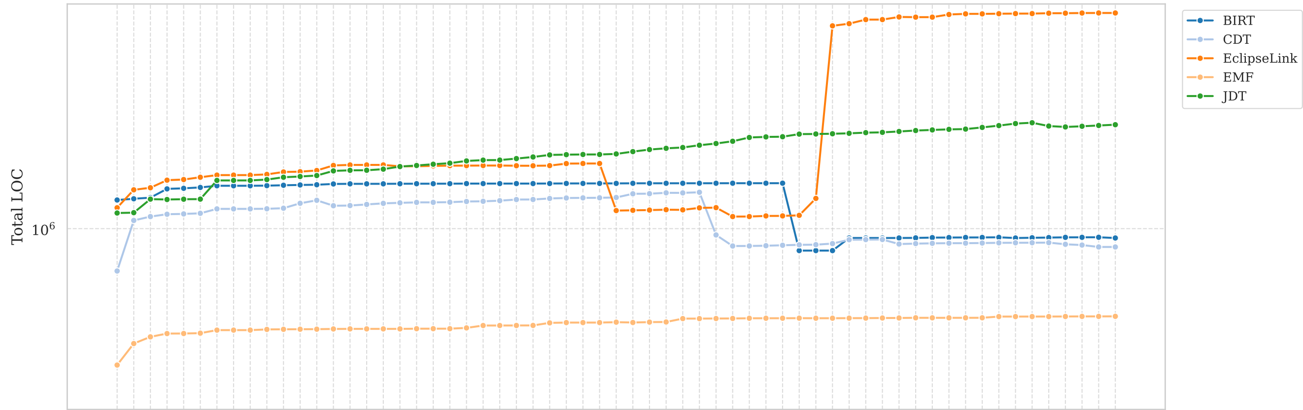
LOC Normalizado (0-100) por Feature (Grandes: Início > 500k LOC) [Base Log]
