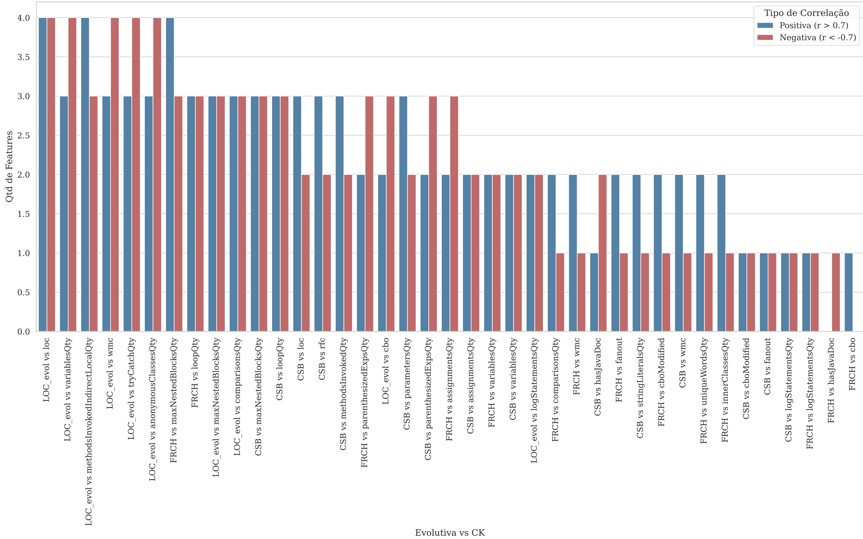
Histograma: Correlações Fortes - Evol vs CK - Empate Técnico (Dif <= 1)
