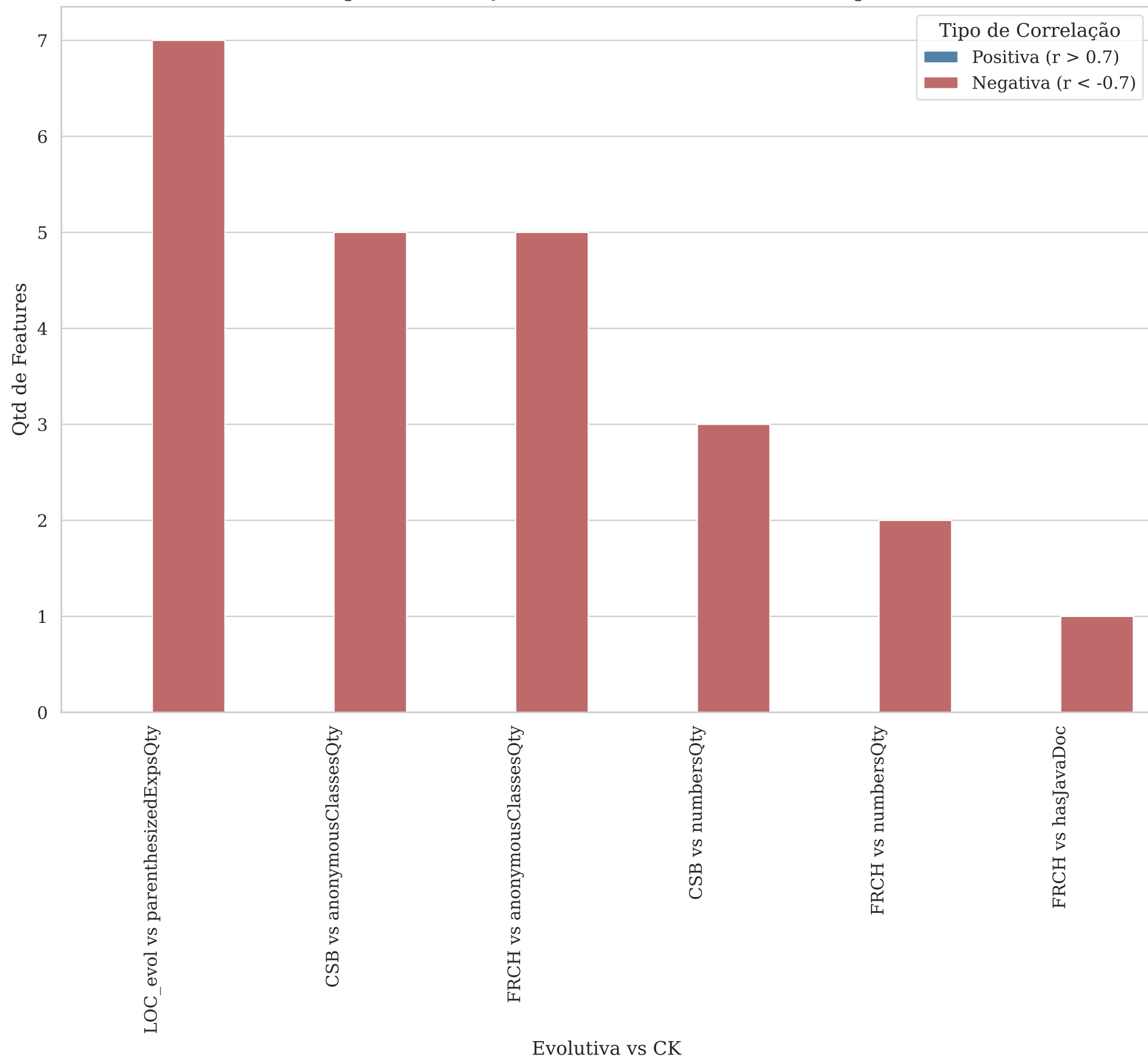
Histograma: Correlações Fortes - Evol vs CK - Somente Negativas
