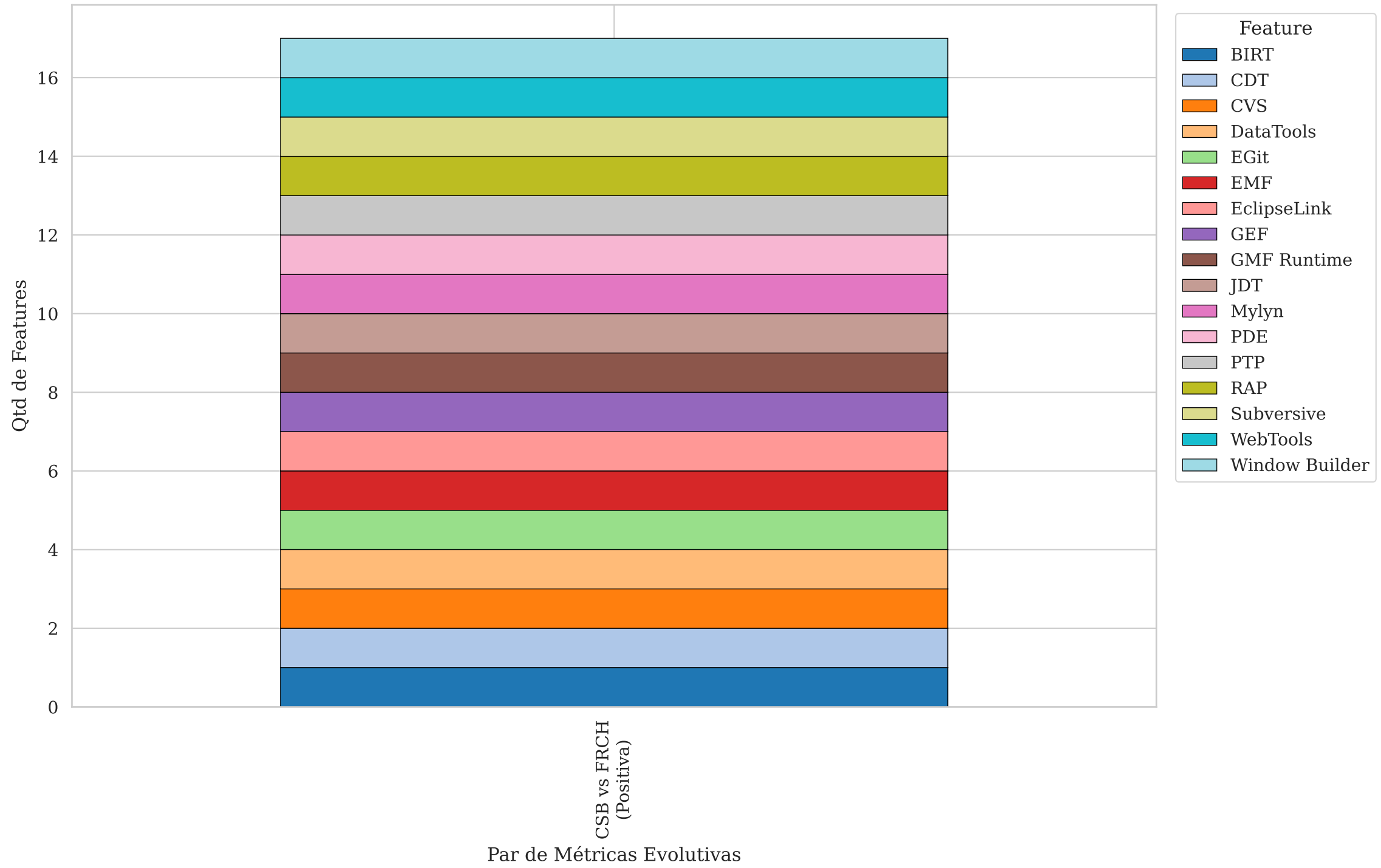
Histograma: Correlações Fortes - Evol vs Evol - Somente Positivas
