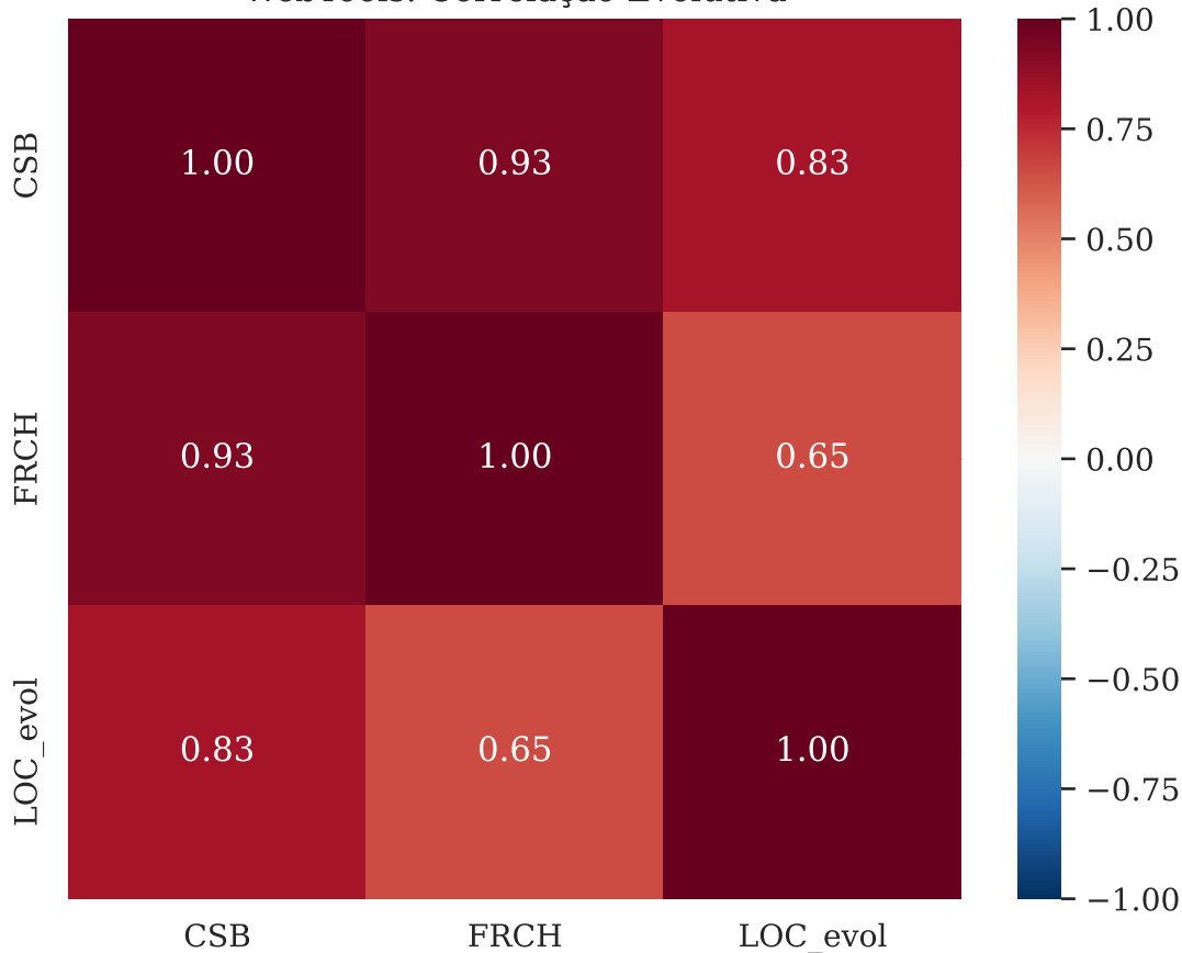
WebTools: Correlação Evolutiva
