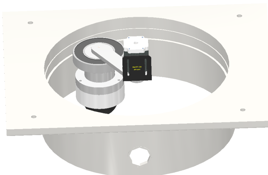
Figura 5.7: Vista del aro de giro y el rodamiento de Ø120 mm.
