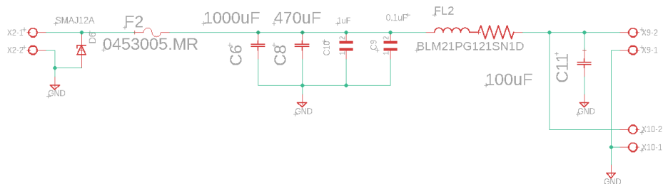
Figura 4.21: Esquemático de la línea de distribución de 12 V.
