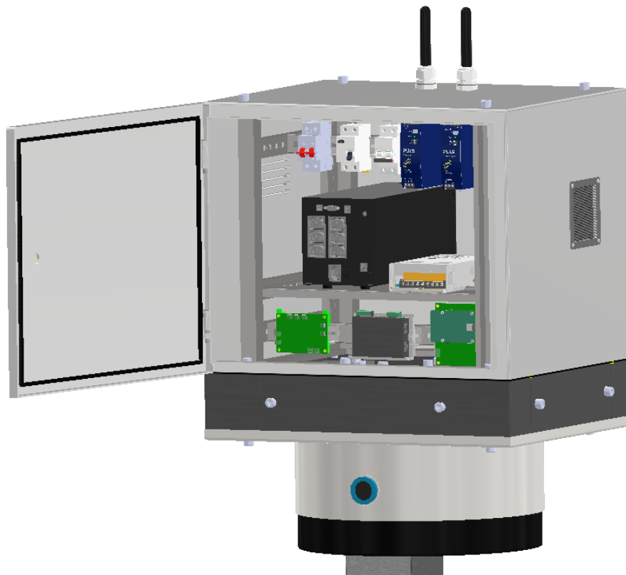
Figura 5.2: Vista general del controlador semafórico propuesto.
