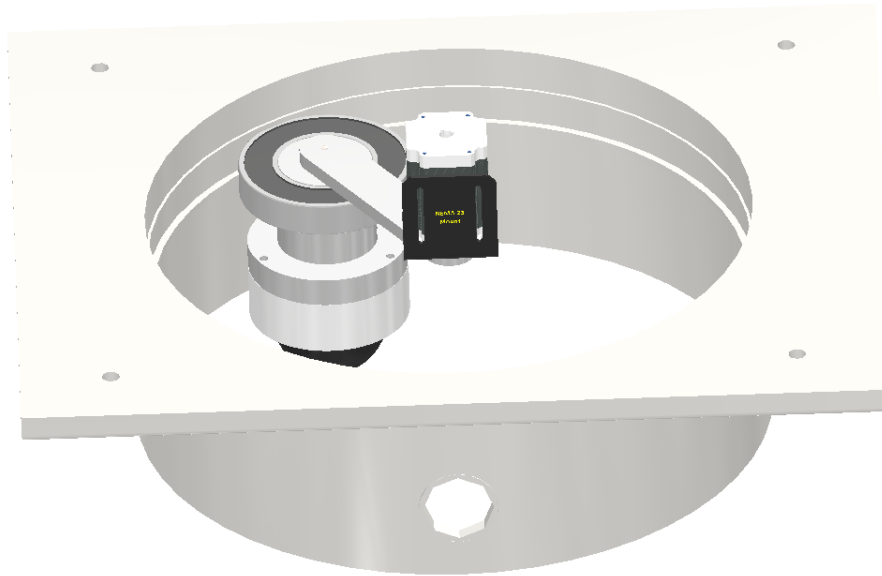
Figura 5.7: Vista del aro de giro y el rodamiento de \varnothing 120 mm.
