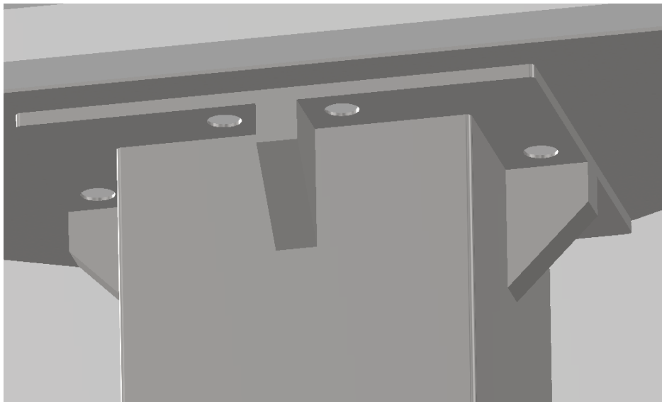
Figura 5.12: Refuerzos triangulares superiores en la conexión gabinete-poste.
