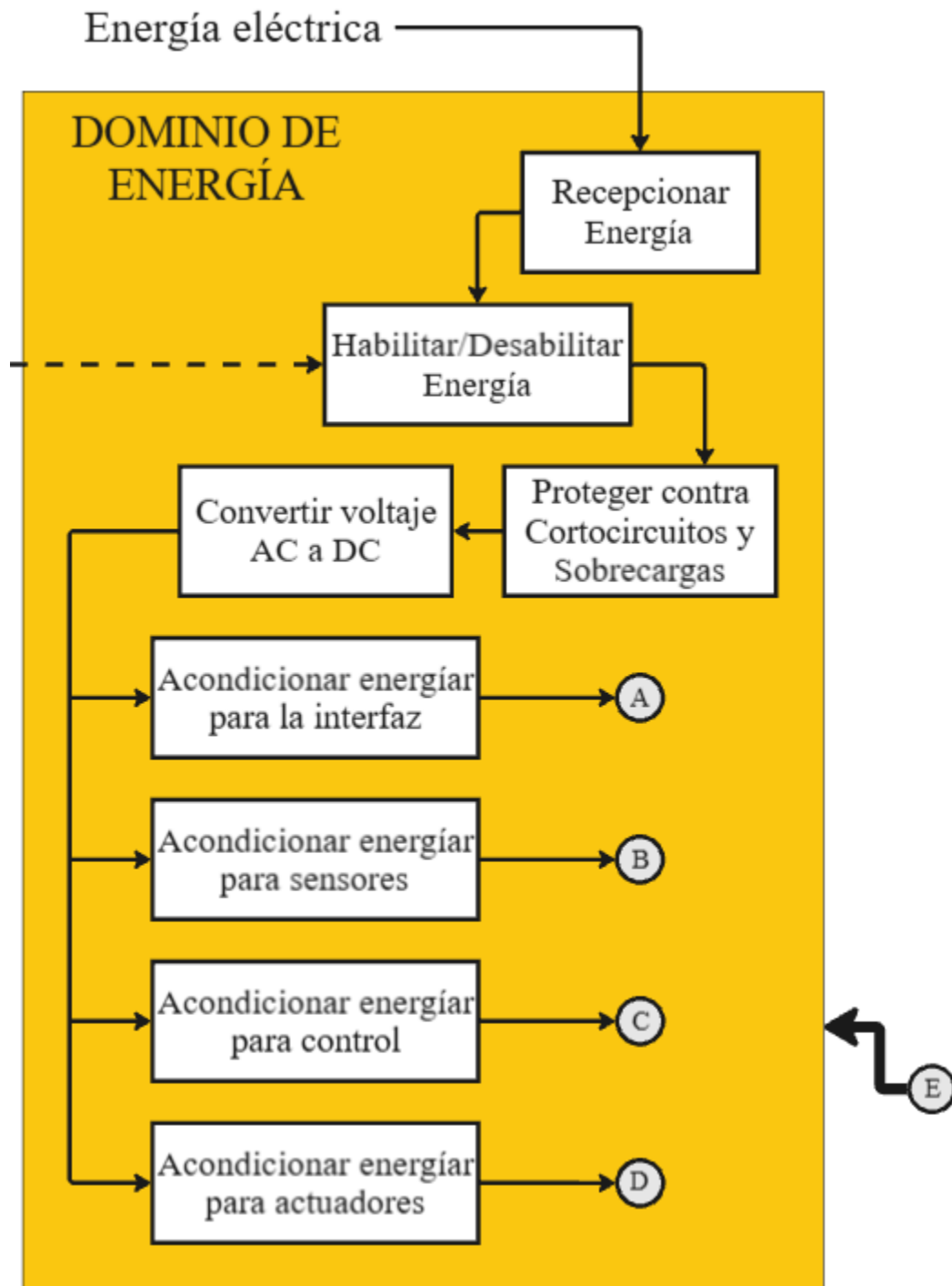
Figura 3.5: Estructura de funciones del dominio de energía.
