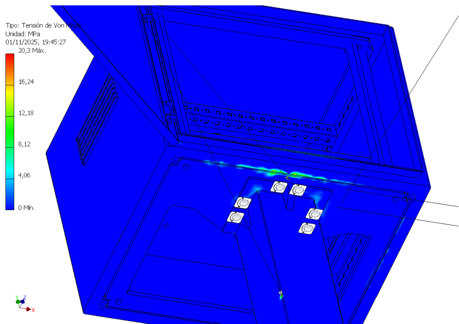
Figura 5.17: Tensión de Von Mises, vista inferior del gabinete. Fuente: Elaboración propia.
