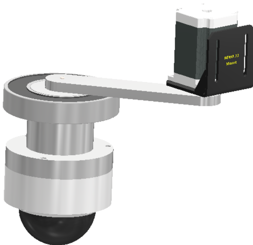
Figura 5.6: Conjunto cámara domo, soporte y biela de transmisión.
