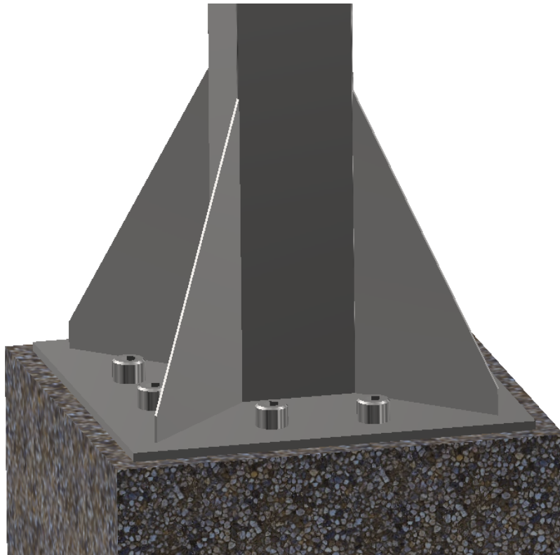
Figura 5.13: Refuerzos triangulares inferiores en la transición poste-zapata.
