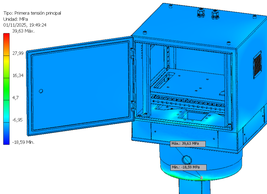
Figura 5.18: Distribución de la primera tensión principal. Fuente: Elaboración propia.
