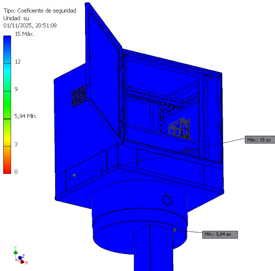
Figura 5.23: Factor de seguridad enfocado en el gabinete. Fuente: Elaboración propia.
