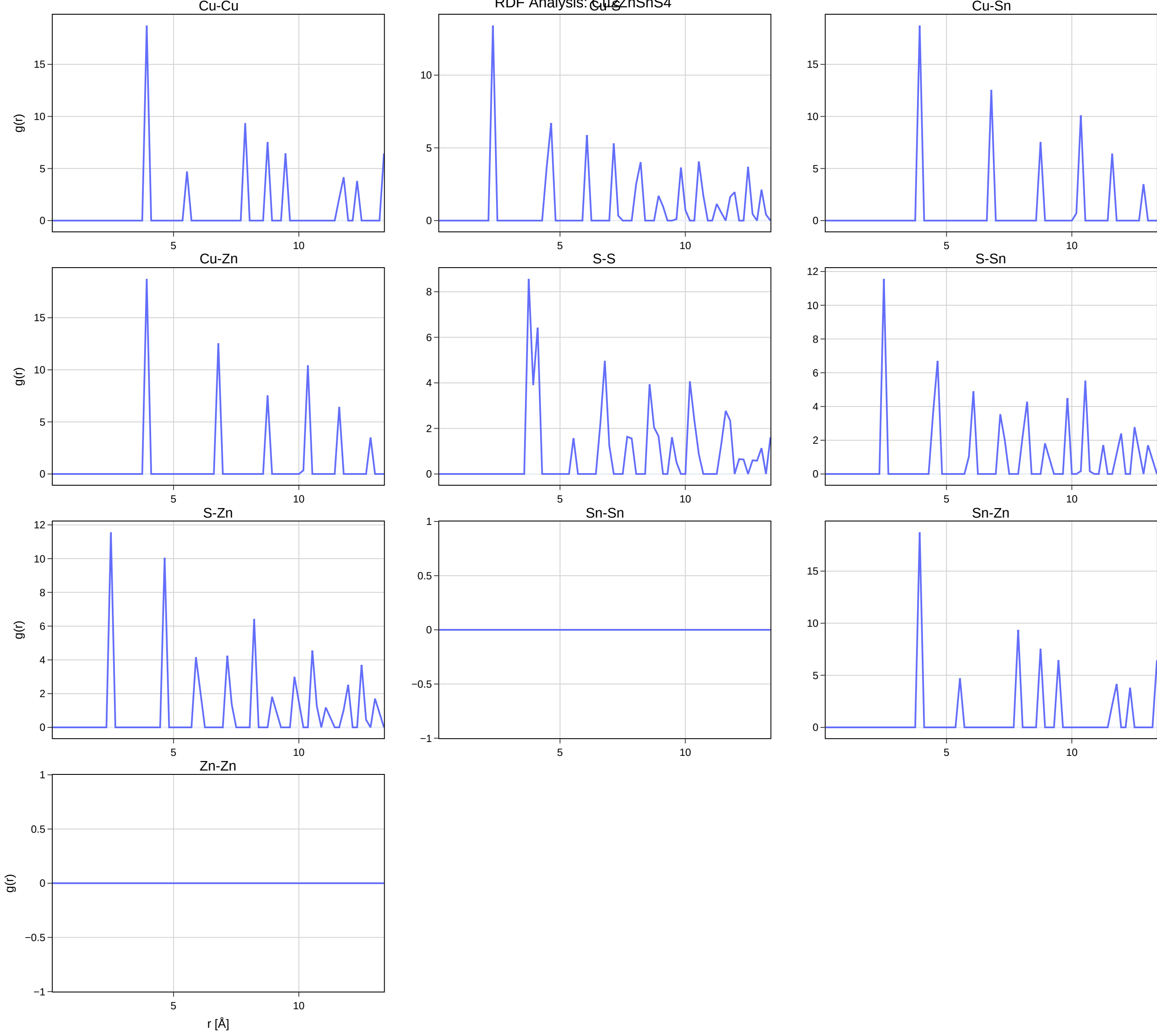
RDF Analysis: Cu 2 ZnSnS 4
