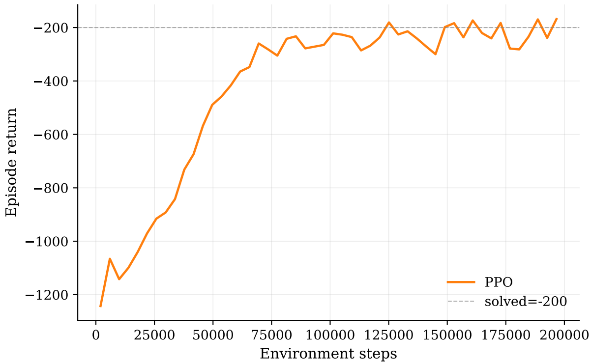
Pendulum-v1
