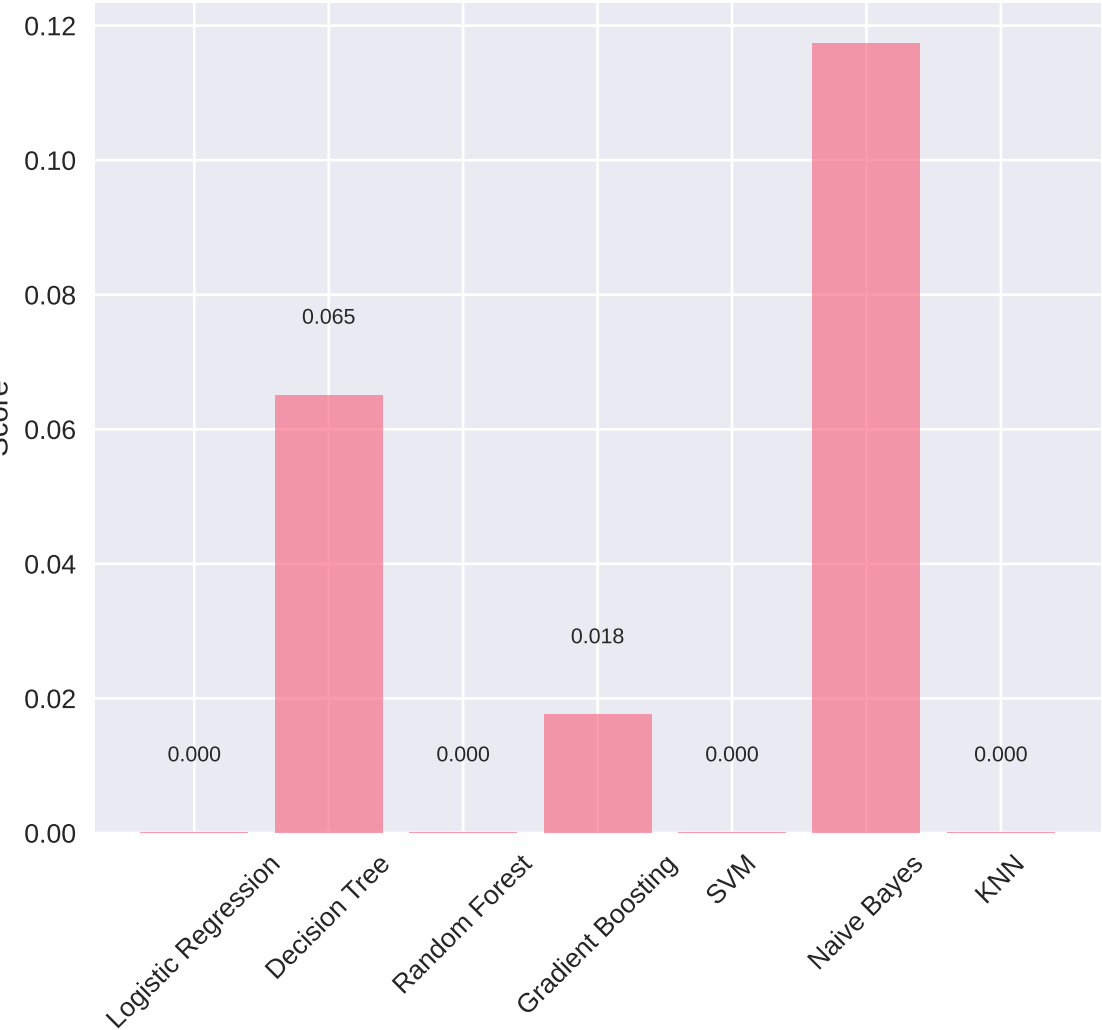
F1 Score
