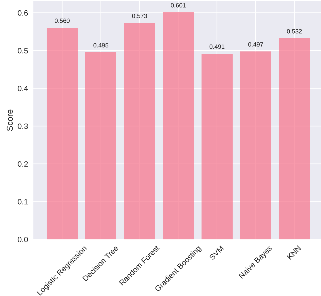
Roc Auc
