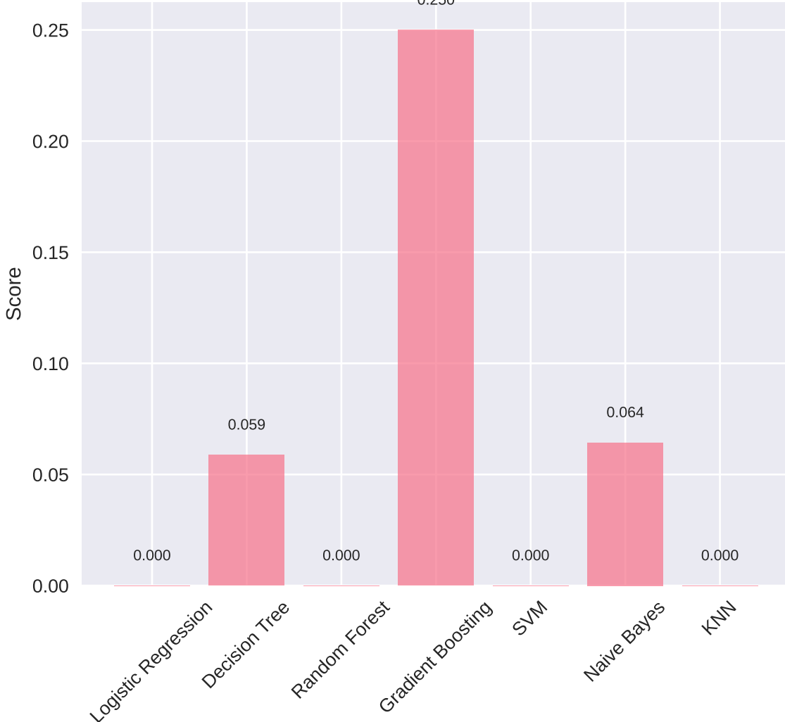
Precision
