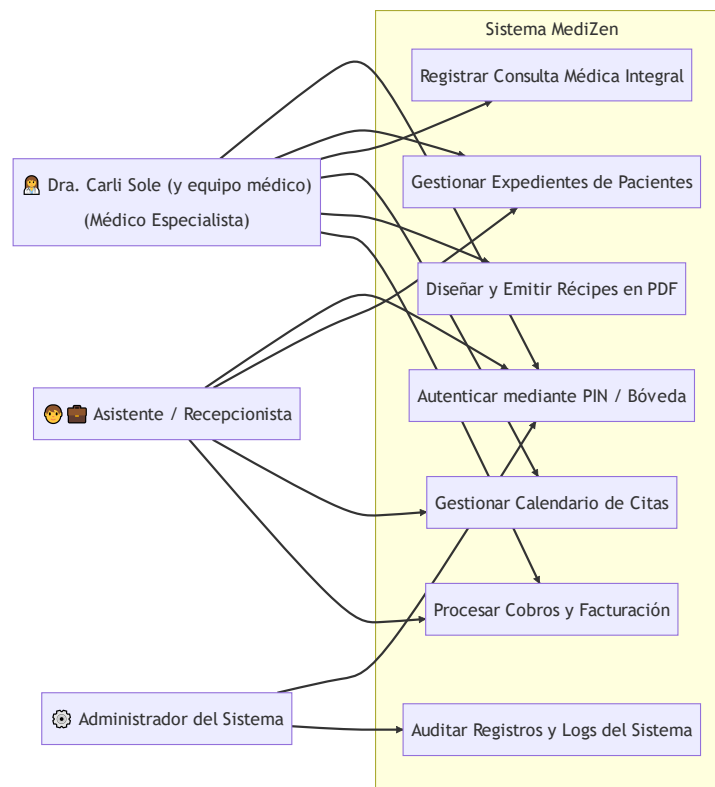
Diagrama de Casos de Uso del Sistema
