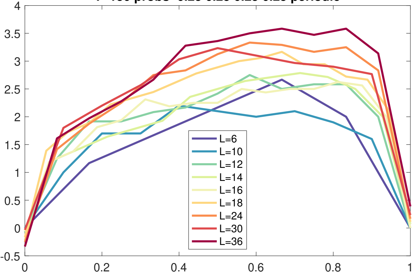
T=150 probs=0.25 0.25 0.25 0.25 periodic
