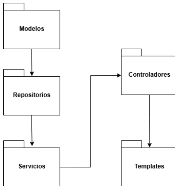
Figura 4. Diagrama de paquetes
