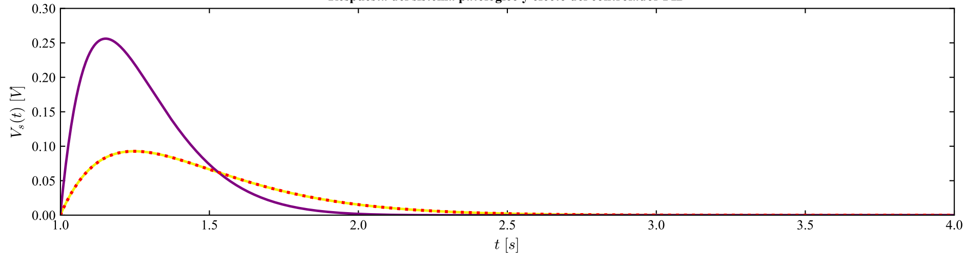
Respuesta del sistema patológico y efecto del controlador PID
