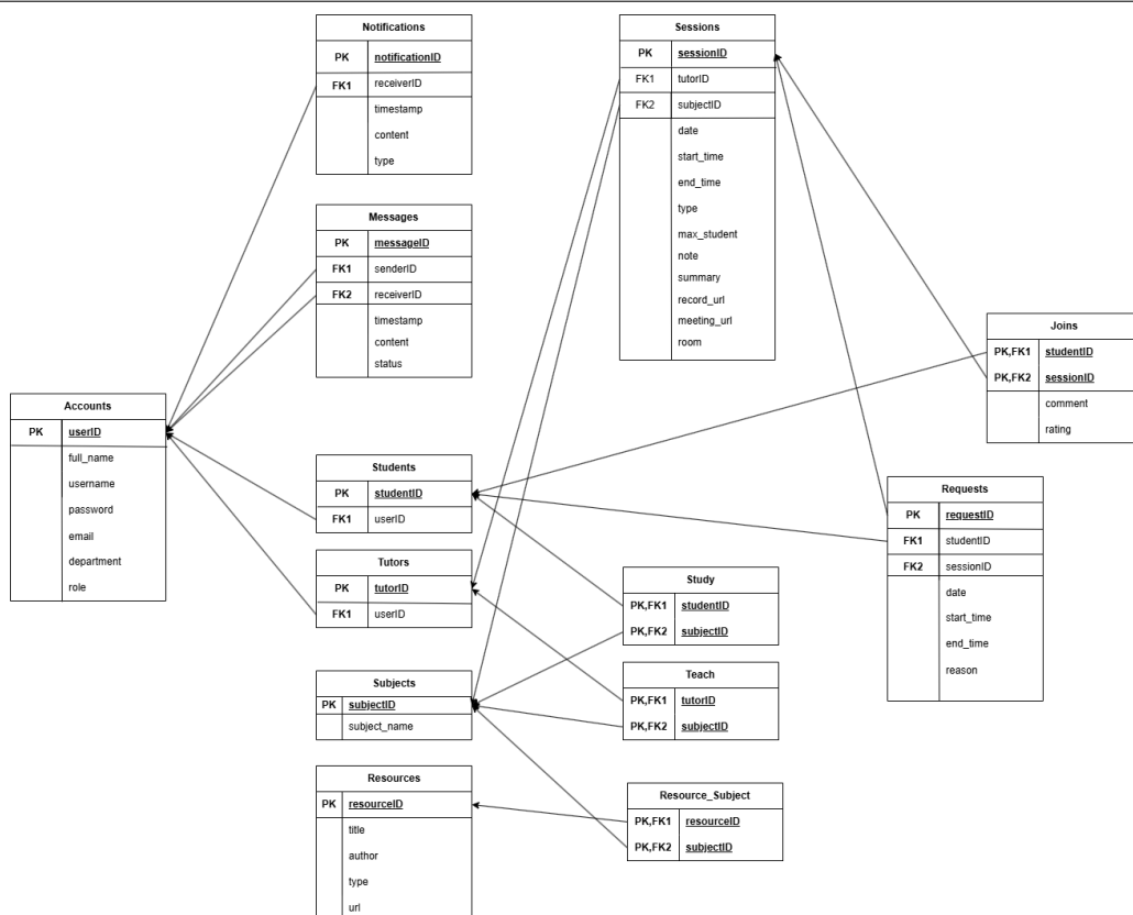
Hình 3.2: Mapping của hệ thống HCMUT_Tutor
