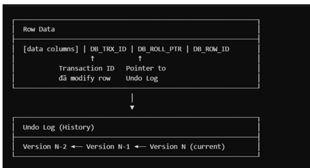
Hình 2.54: Minh họa cơ chế MVCC
