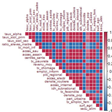
Matrice de corrélation des 23 indicateurs
