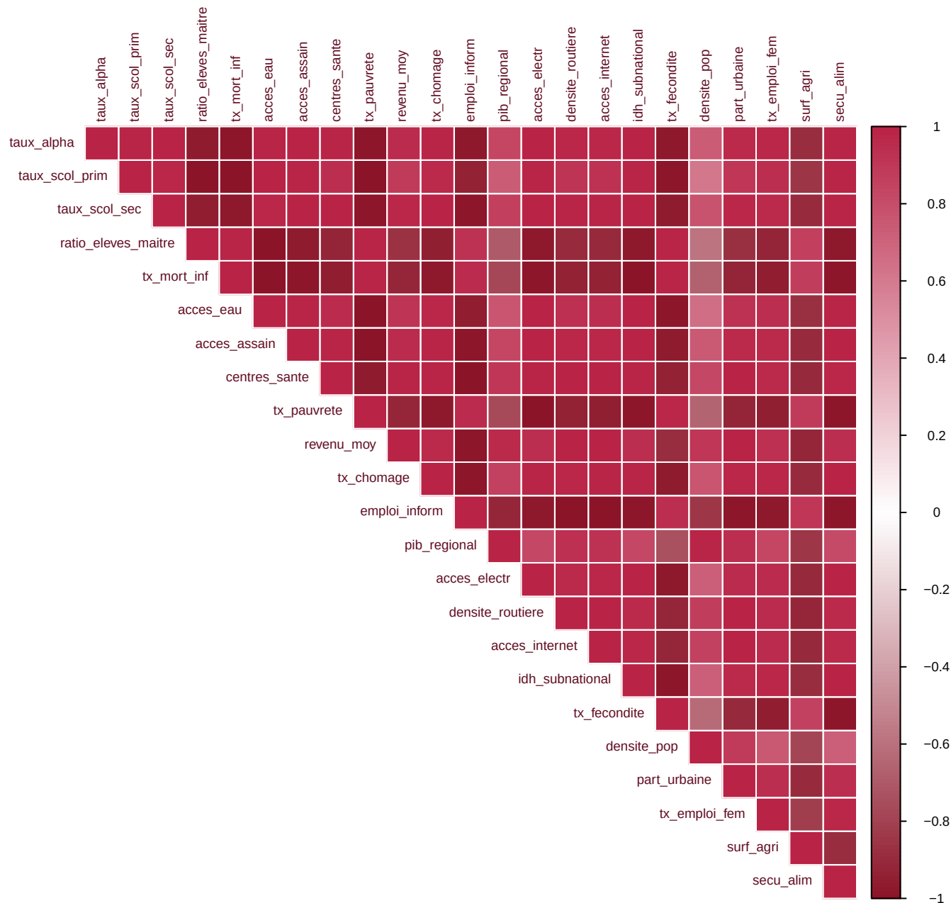
Matrice de corrélation de Pearson — 23 indicateurs
