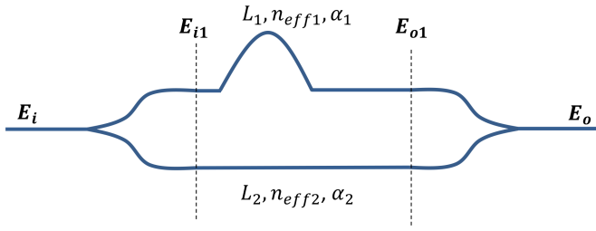
Fig. 4. Imbalanced MZI.
