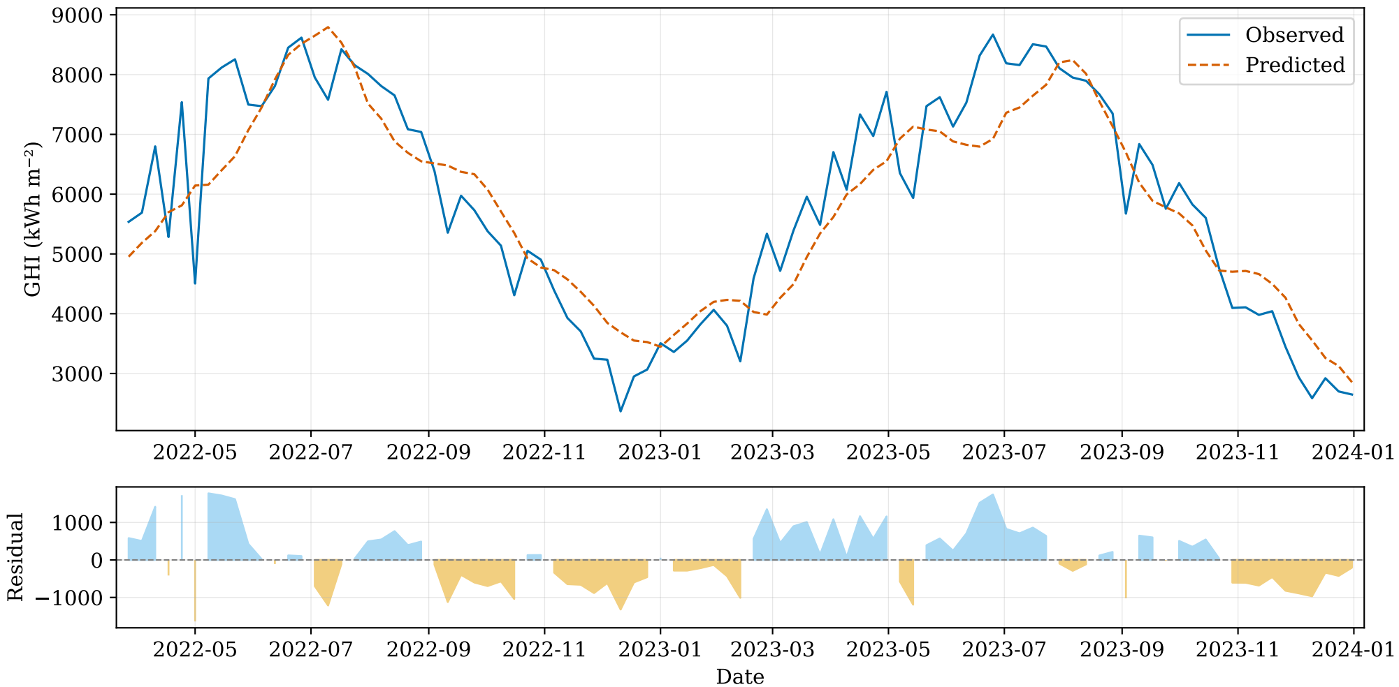
Predictions - GRU
