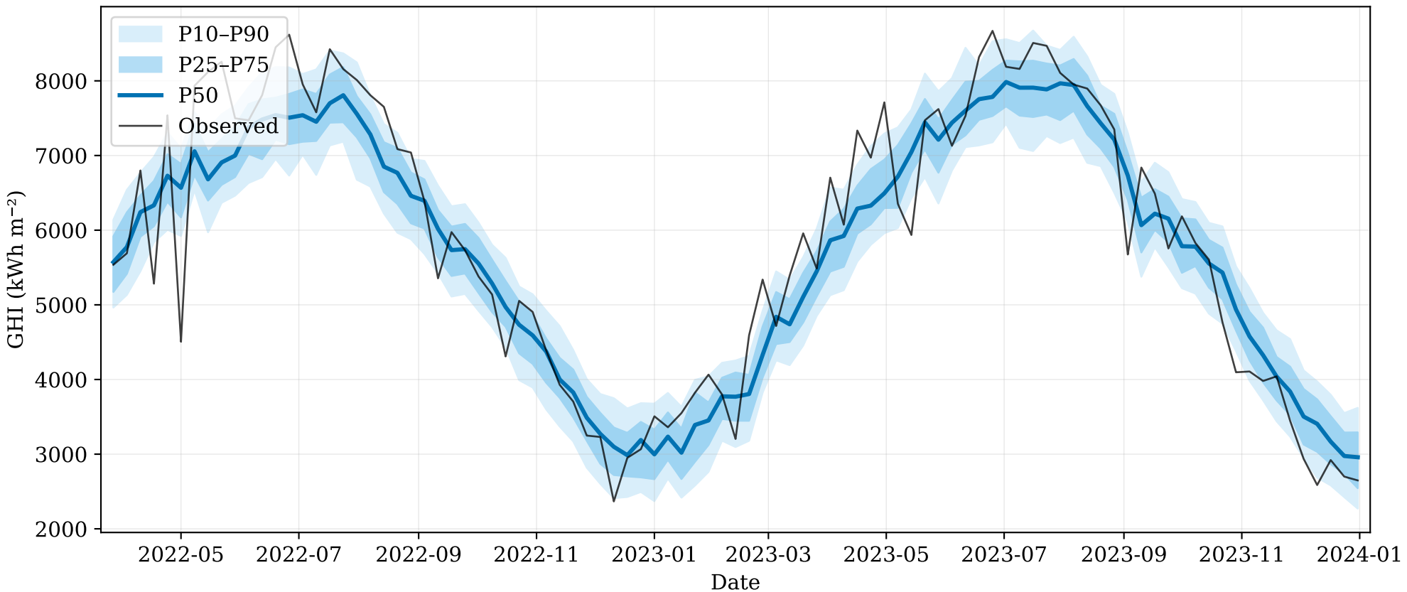
Fan Chart - TRANSFORMER
