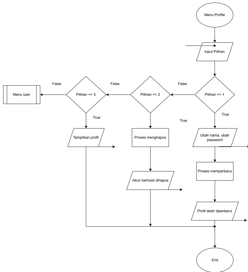
Gambar 2.16 Flowchart Profil
