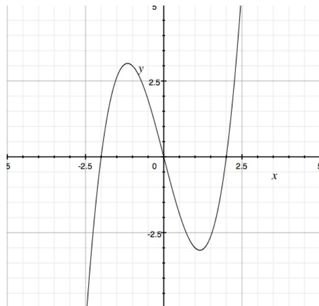
Hình 2.1: An example graph
