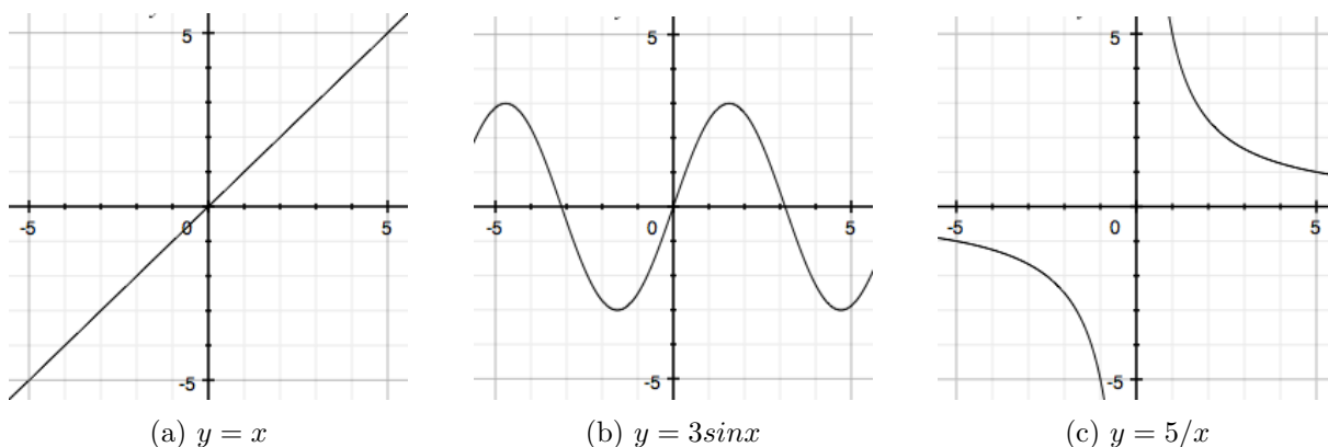
Hình 3.1: Three simple graphs
