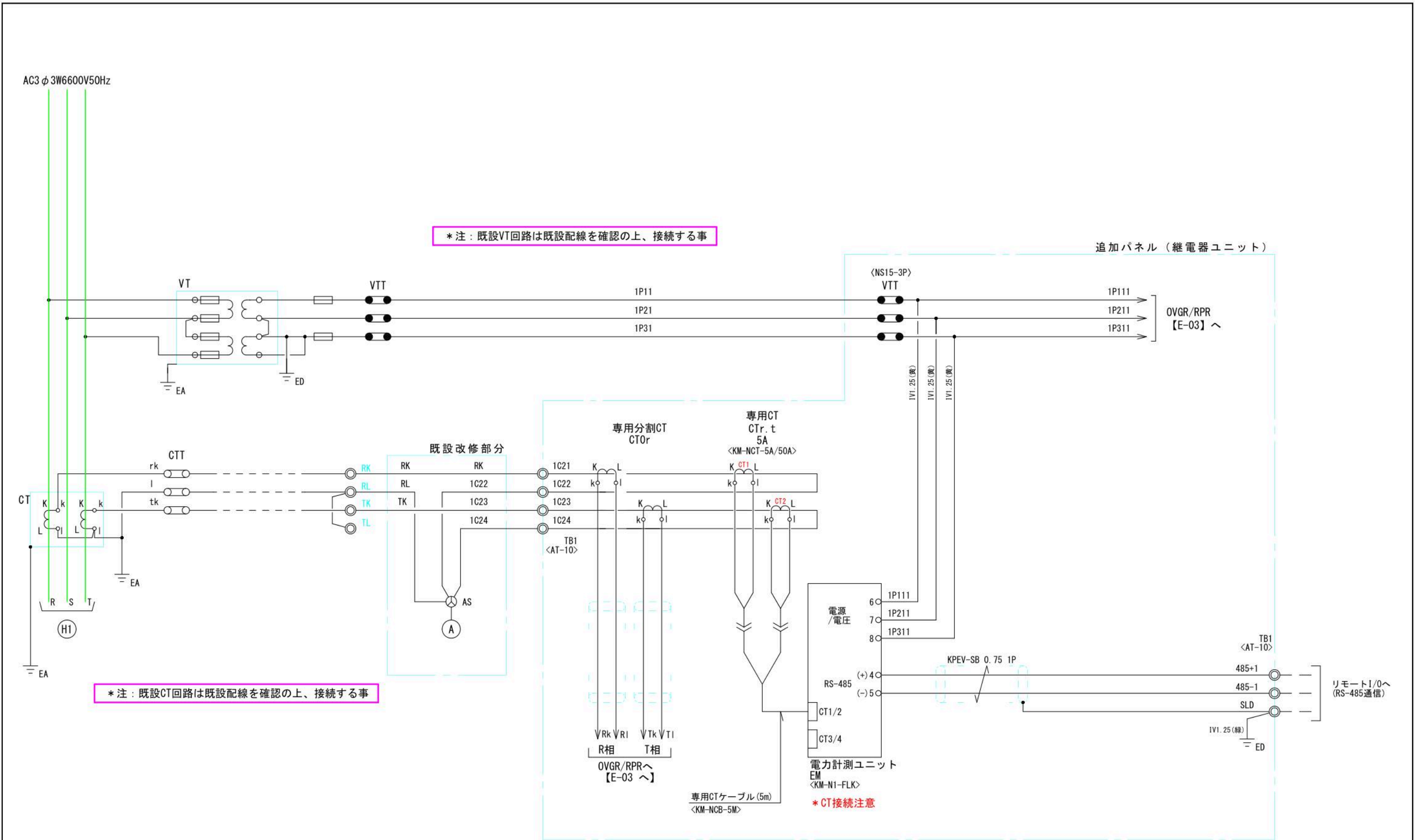
受電VT・CT回路 参考図
