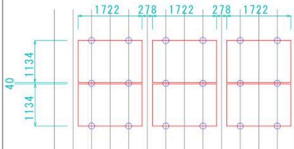
モジュール取り付け詳細図
