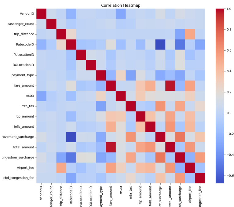
Hình 7: Ma trận tương quan giữa các biến số
