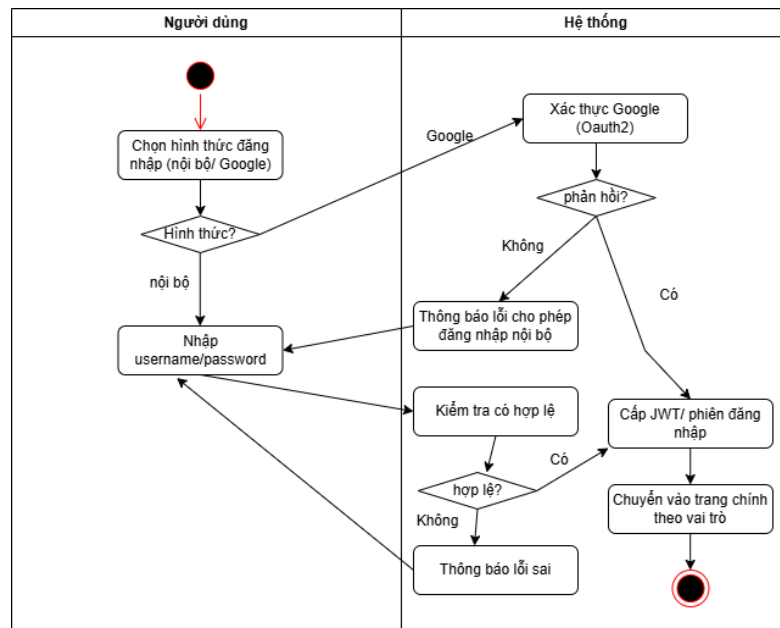
Hình 4. Sơ đồ hoạt động uc đăng nhập
