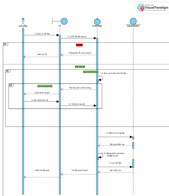
Hình 12. Sơ đồ tuần tự uc nhập dữ liệu CSV, hình ảnh
