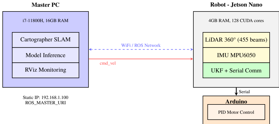
Hình 3.6. Kiến trúc hệ thống robot hoàn chỉnh
