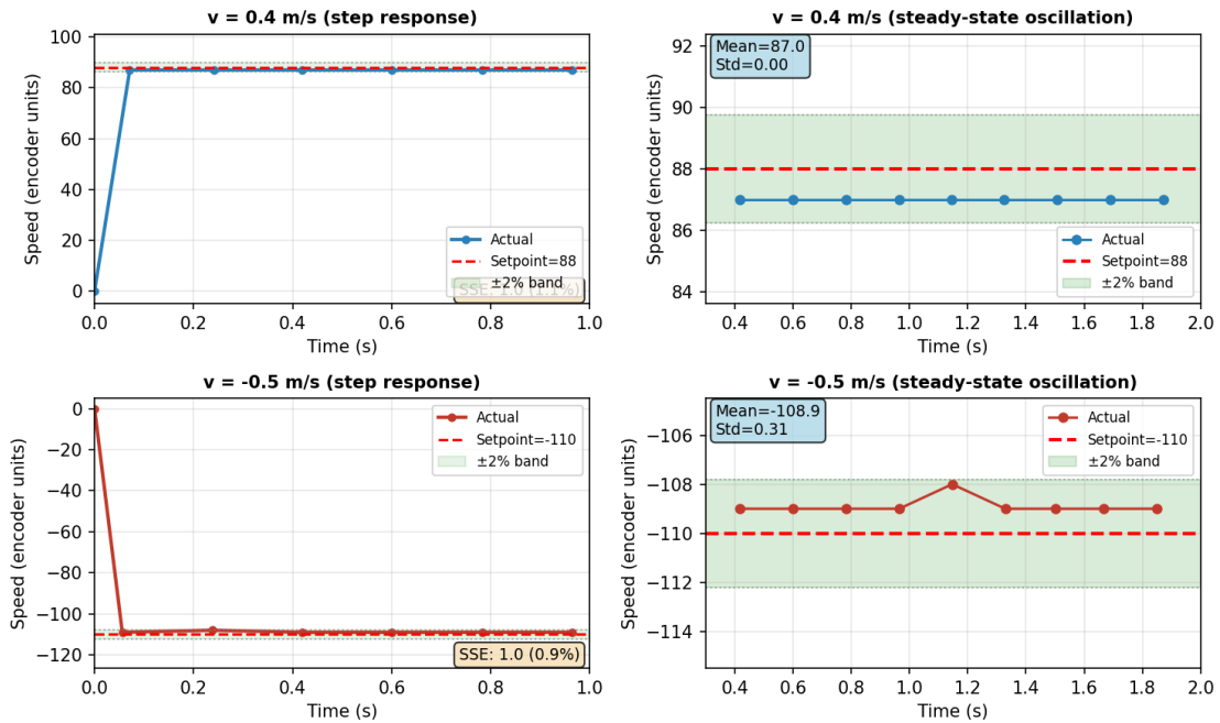
Hình 3.5. Đáp ứng step response của bộ PID. Hàng trên: v = 0.4 m/s (88 units), hàng dưới: v = -0.5 m/s (-110 units). Cột trái: step response 0-1s, cột phải: zoom vào vùng steady-state (0.3-2s) để thấy dao động quanh setpoint.
