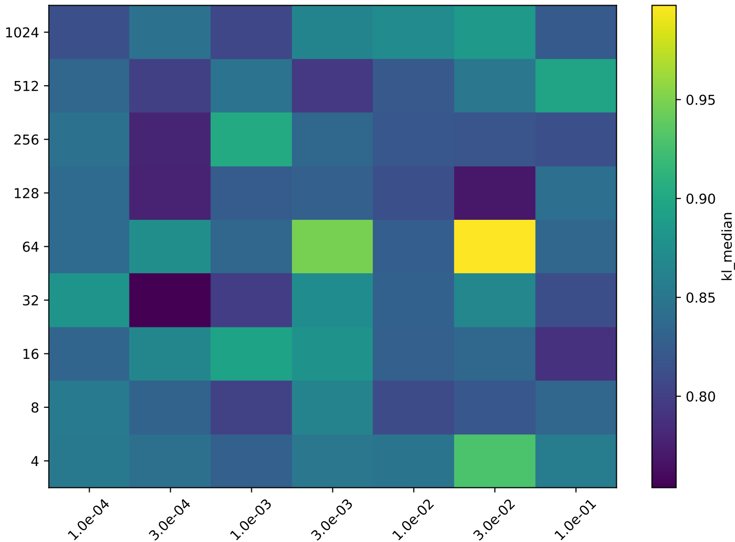
KL Median (lambda=0.0)
