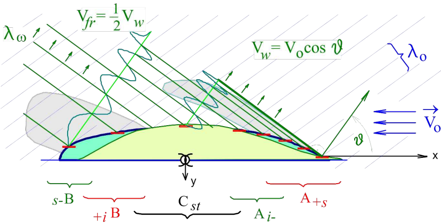
Рис. 17. Волнообразование , как процесс отражения волн от поверхности корпуса корабля. В зонах A_{+s} и s-B происходит рост гребня трохoidalной волны, неспособной отойти от корпуса судна.
