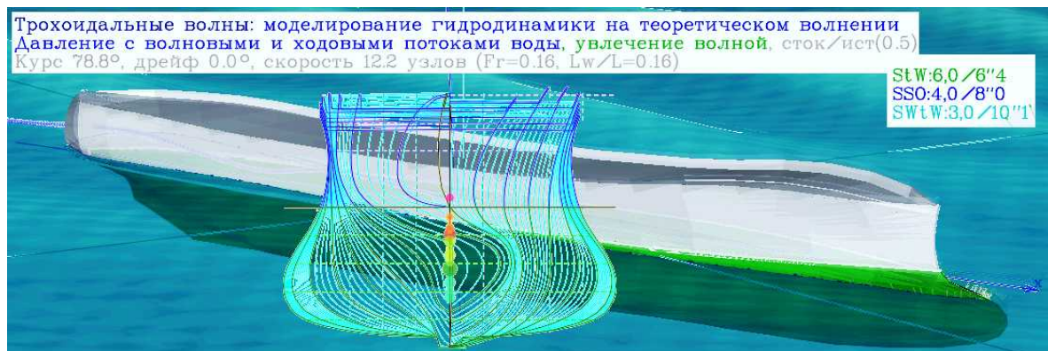
Рис. 16. Универсальное транспортное судно (A1203-Univer-86) с завалом борта на уровне твиндеков под верхней палубой, представленное руководителю, профессору Александра Николаевичу Холодильнику в качестве основного результата мореходных испытаний в опытовом бассейне в ЛКИ в 1985 году. Аперриодический режим бортовой качки при нулевой начальной остойчивости; и плавность килевой качки предотвращает заливаемость верхней носовой палубы, несмотря на снижение высоты форштевня, устроенного для предотвращения силового захвата корпуса встречной волной.
