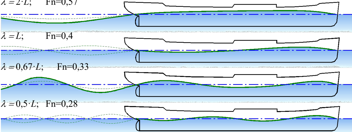
Рис. 13. Характерные режимы волнообразования при различных скоростях движения судна V \approx 1,25 \cdot \sqrt{(\lambda/L) \cdot L} = 1,25 \cdot \sqrt{\lambda} \text{ [м/с]} . Иллюстрируется интерференция корабельных волн, условно зарождающихся на форштевне и ахтерштевне
