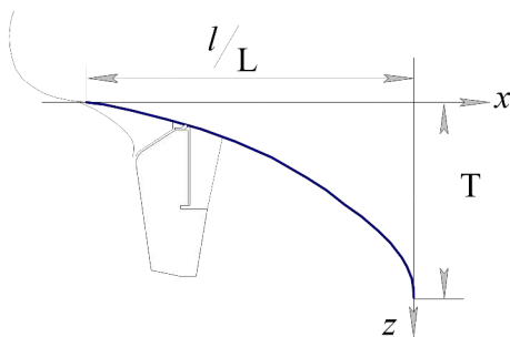
Рис. 10 Аппроксимация кормового подзора частью от четвертинки эллипса.
