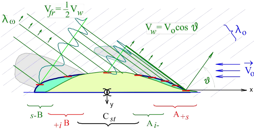
Рис. 17. Волнообразование , как процесс отражения волн от поверхности корпуса корабля. В зонах A_{+s} и s-B происходит рост гребня трохoidalной волны, неспособной оторваться от корпуса судна.
