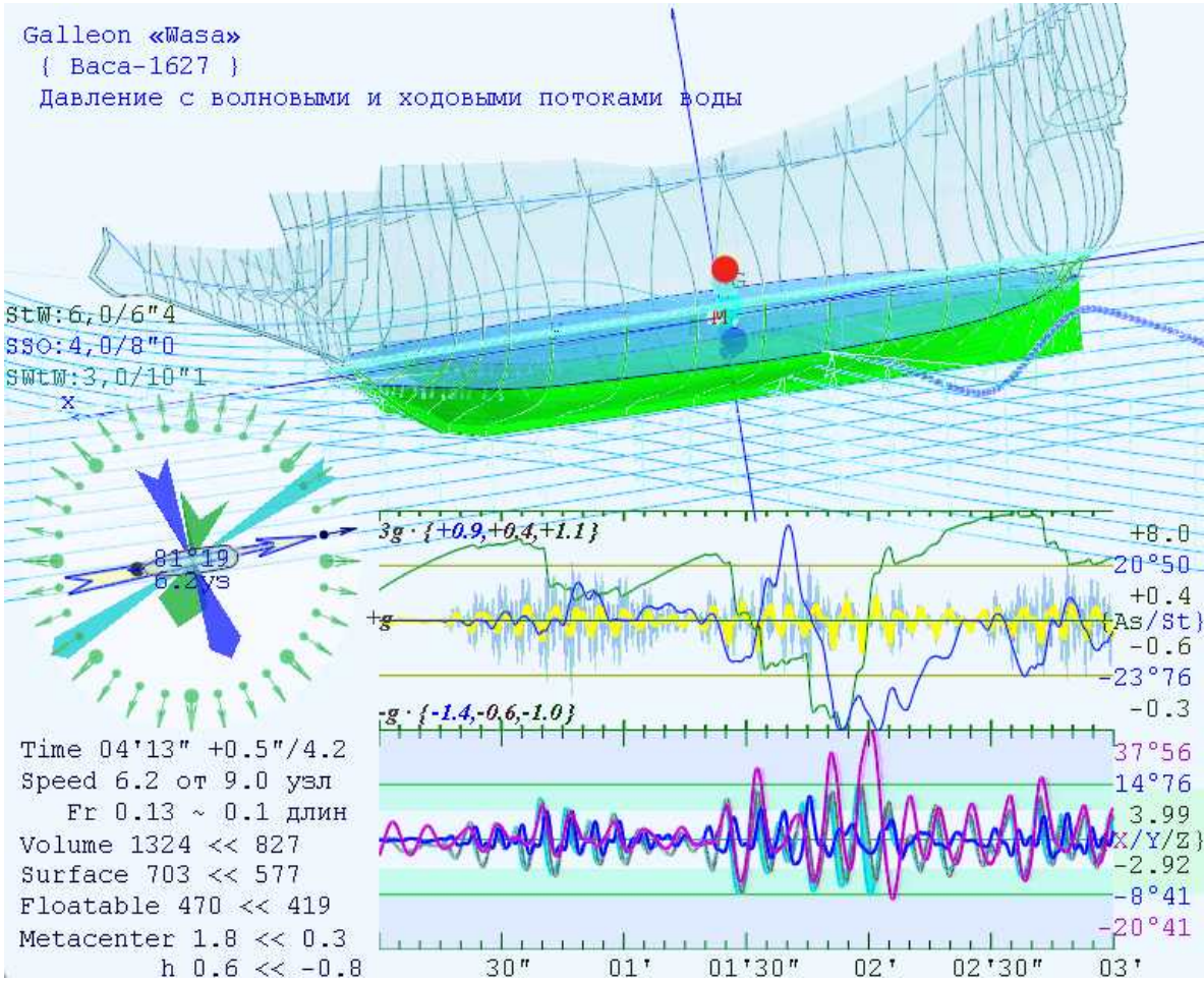
Рис. 23. Ход вычислительного эксперимента в окне для представления гидромеханики ко-рабля. Вертикальная качка превышает 7 метров. Сильное рыскание и дрейф по курсу возникает в моменты экстремальной бортовой качки. Внизу графики бортовой X, килевой Y и вертикальной Z качки с масштабной шкалой справа. На левой шкале верх-них графиков масштаб для кривых вертикальных ускорений.
