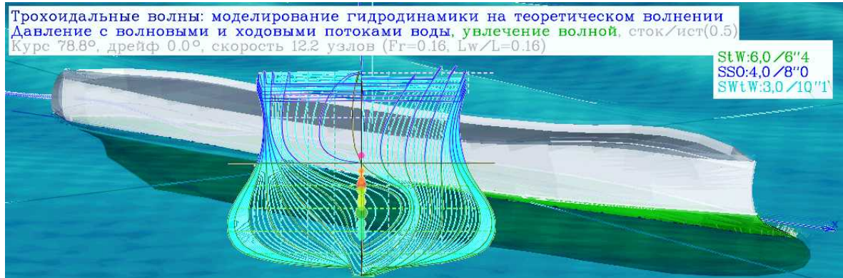
Рис. 16. Универсальное транспортное судно (А1203-Univer-86) с завалом борта на уровне твиндеков под верхней палубой, представленное руководителю, профессору Александра Николаевичу Холодилину в качестве основного результата мореходных испытаний в опытовом бассейне в ЛКИ в 1985 году. Аперриодический режим бортовой качки при нулевой начальной остойчивости; и плавность килевой качки предотвращает заливаемость верхней носовой палубы, несмотря на снижение высоты форштевня, устроенного для предотвращения силового захвата корпуса встречной волной.
