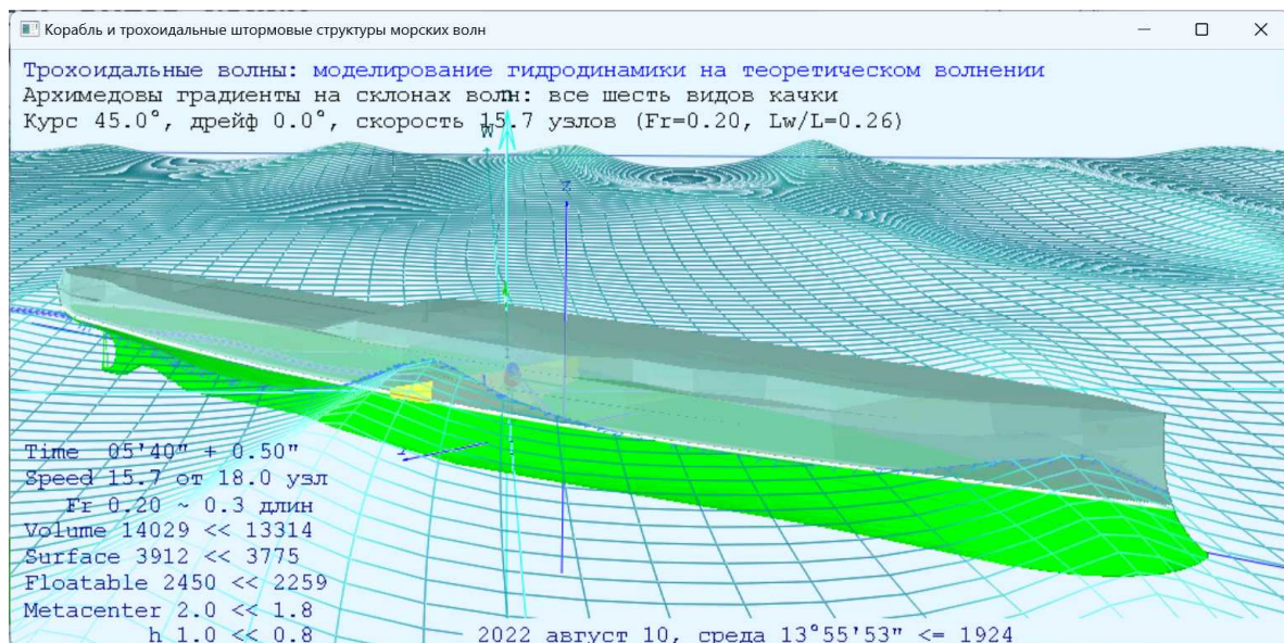
Рис. 24. «Корабль и трохойдальные штормовые структуры морских волн» – воспроизведение морского волнения в опытовых изысканиях мореходности корабля в условиях штормового плавания. Контурные прорисовки профилей трохойдальных волн большой крутизны выполняются на фоне соизмеримой по высоте длиннопериодной зыби.
