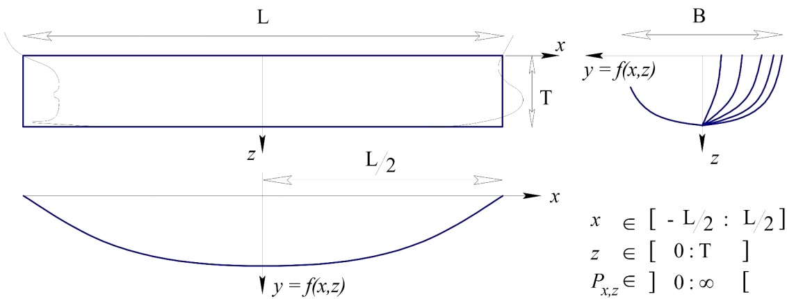
Рис. 6. Область определения и размерения аналитической модели симметричного относительно мидельшпангоута корпуса корабля – КПО - корпус параболических обводов.
