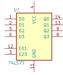
74LS77
