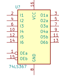
74LS367
