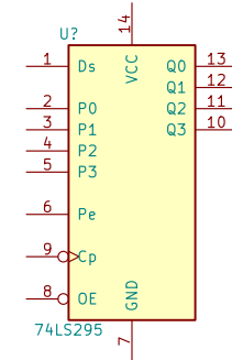
74LS295
