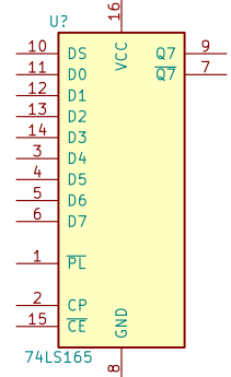
74LS165
