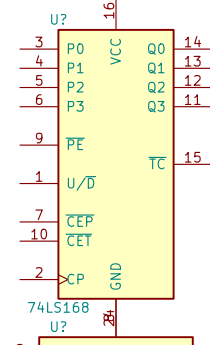
74LS168
