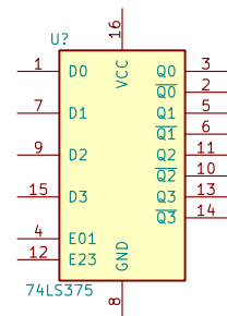
74LS375
