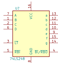
74LS248
