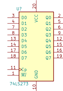
74LS273
