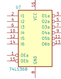
74LS368
