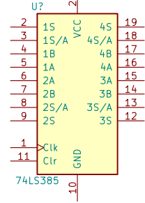
74LS385
