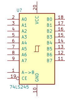
74LS245
