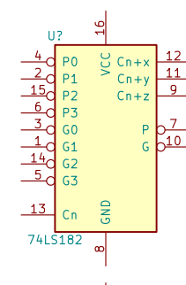
74LS182
