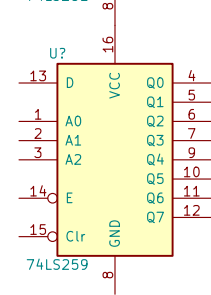
74LS259
