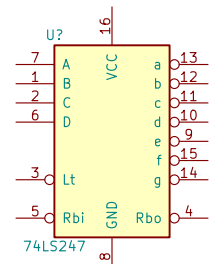
74LS247
