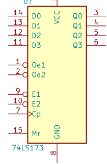
74LS173
