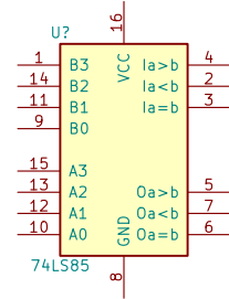
74LS85
