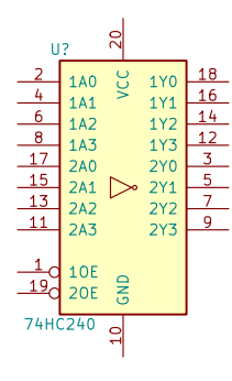
74HC240
