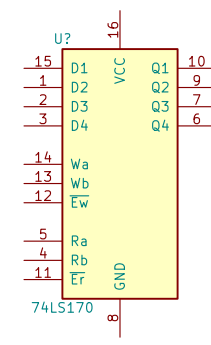
74LS170
