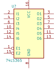
74LS365
