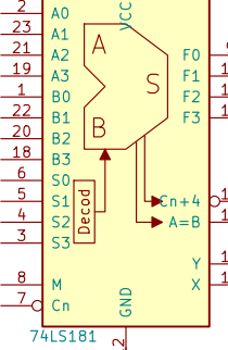
74LS181
