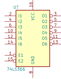
74LS366
