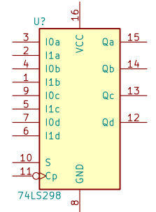
74LS298
