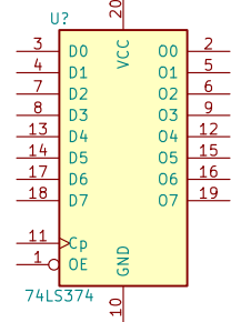
74LS374
