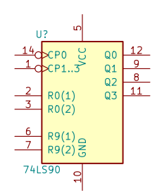
74LS90
