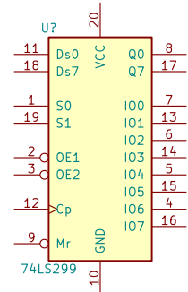
74LS299
