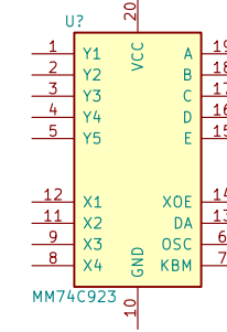
MM74C923
