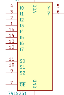
74LS251
