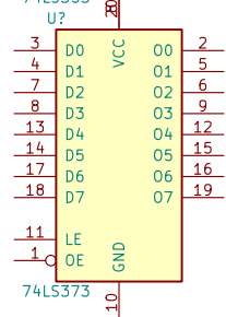
74LS373
