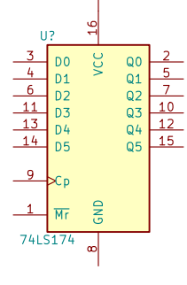
74LS174
