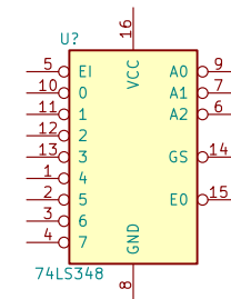
74LS348
