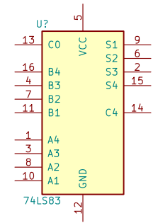
74LS83
