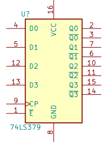
74LS379
