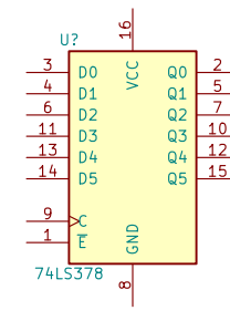
74LS378
