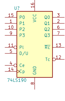
74LS190
