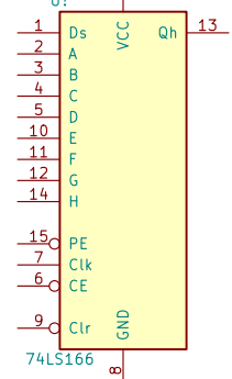
74LS166
