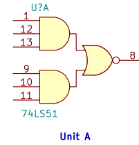
74LS51
