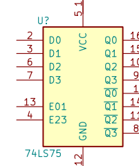
74LS75
