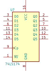
74LS174
