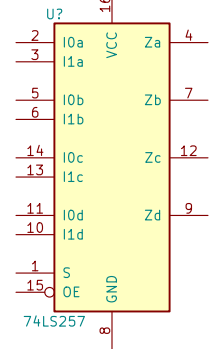
74LS257
