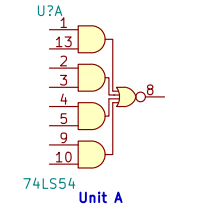
74LS54
