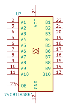
74CBTLV3861
