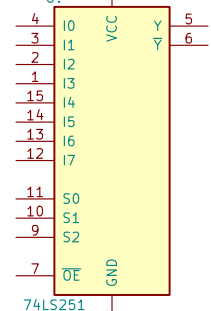
74LS251
