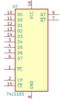
74LS165
