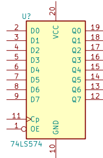
74LS574
