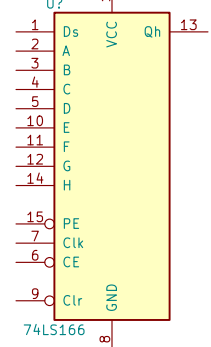
74LS166
