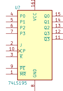
74LS195
