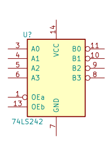
74LS242
