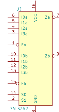
74LS352
