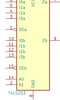
74LS253
