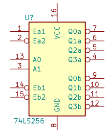
74LS256
