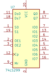
74LS299
