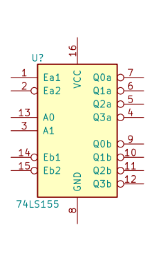
74LS155
