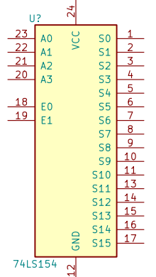
74LS154
