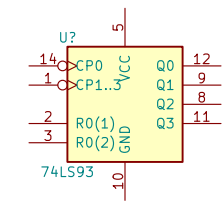
74LS93
