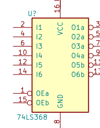
74LS368
