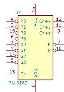
74LS182
