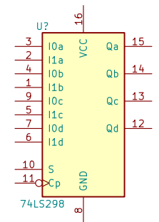
74LS298
