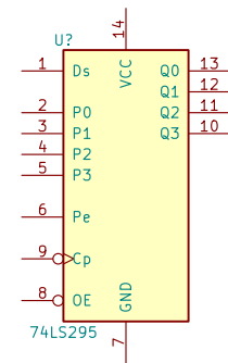
74LS295
