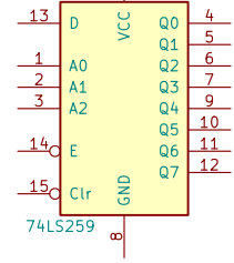
74LS259
