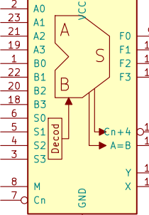
74LS181
