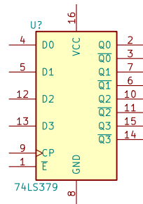
74LS379
