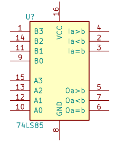
74LS85
