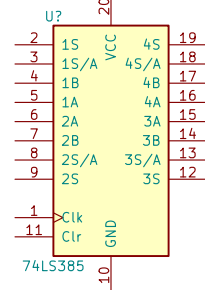
74LS385
