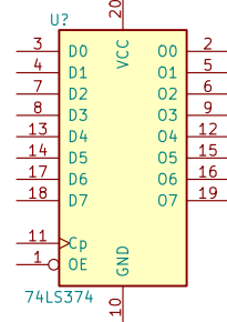
74LS374
