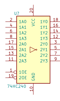
74HC240
