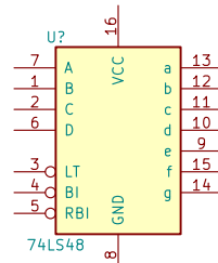
74LS48
