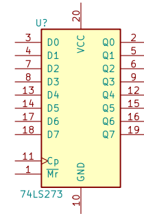
74LS273
