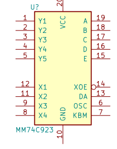
MM74C923
