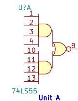
74LS55
