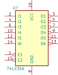
74LS366
