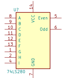
74LS280
