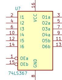
74LS367
