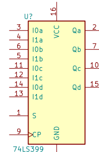
74LS399
