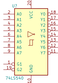
74LS540
