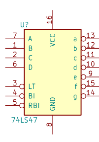
74LS47
