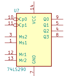
74LS290
