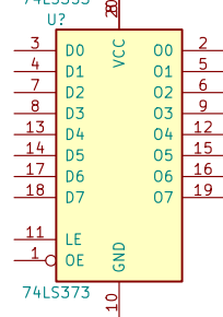
74LS373
