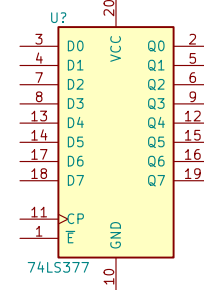
74LS377
