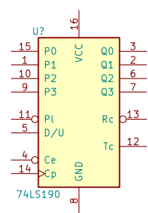
74LS190
