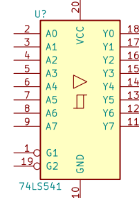
74LS541
