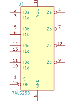
74LS258
