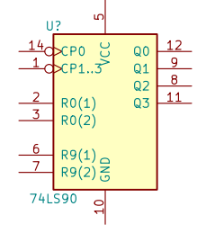
74LS90
