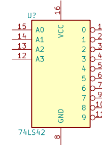
74LS42
