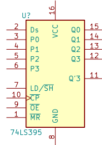
74LS395
