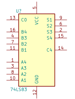
74LS83
