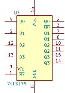
74LS175
