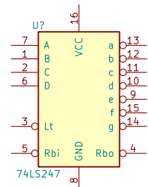
74LS247
