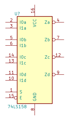
74LS158
