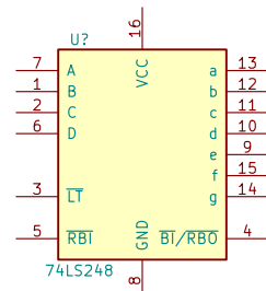
74LS248
