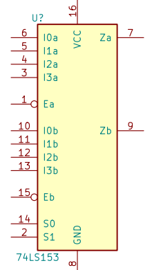
74LS153
