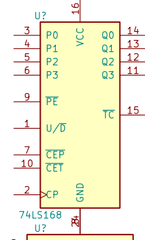
74LS168
