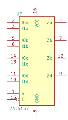
74LS157
