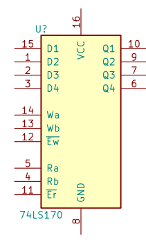
74LS170
