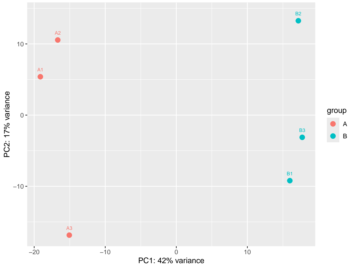
PCA plot
