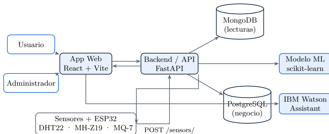
Figura 1: Arquitectura: usuarios y administrador operan la app web, que consume el backend FastAPI; éste persiste en MongoDB/PostgreSQL, invoca el modelo ML e IBM Watson, y recibe la telemetría del hardware IoT.
