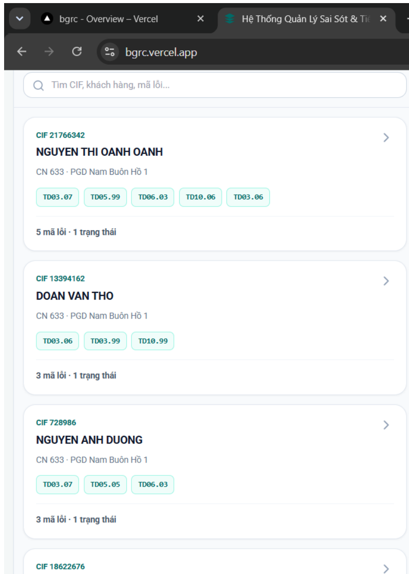
Hình 3 - Giao diện mobile gom CIF, khách hàng, đơn vị, mã lỗi và trạng thái trong từng thẻ.
