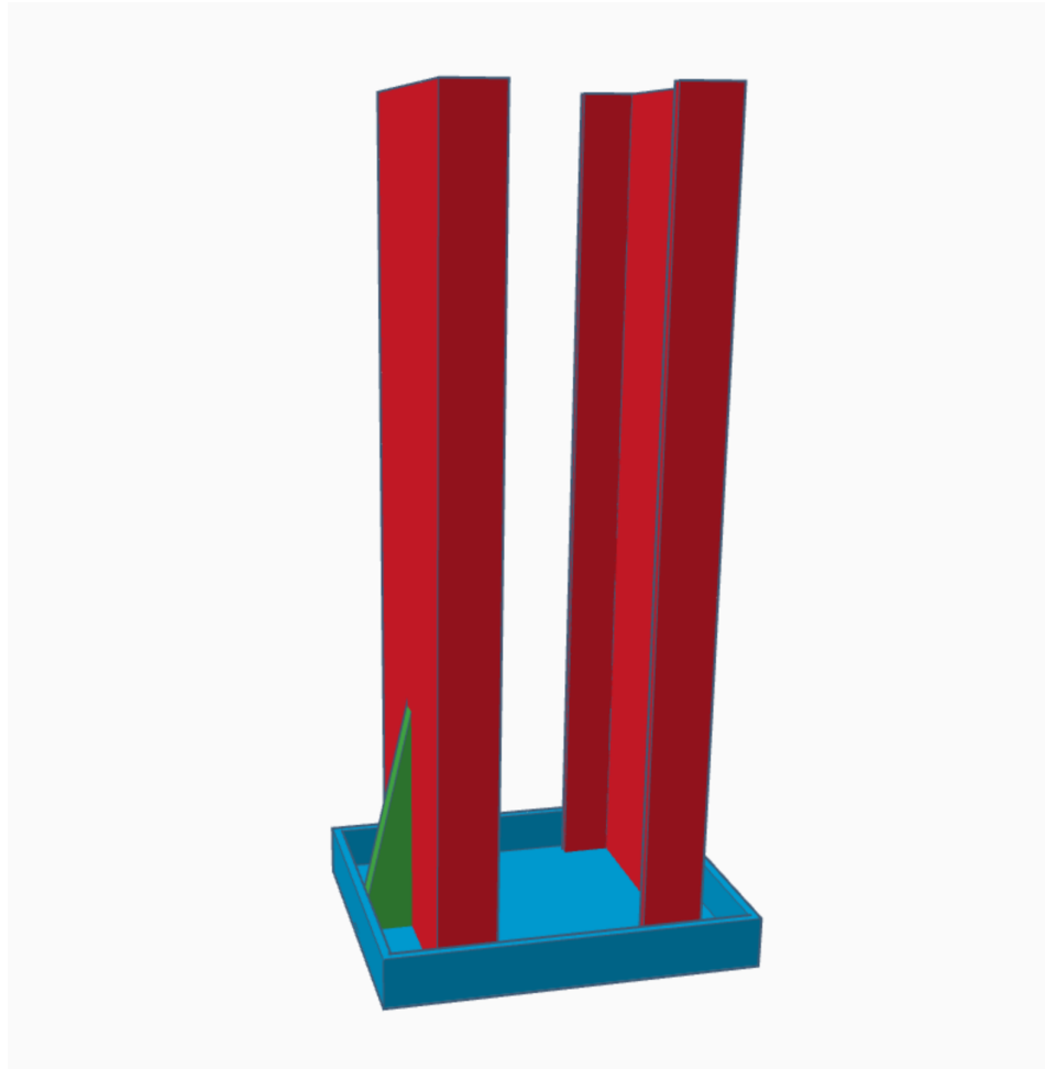
Figura 1: Diseño 3D realizado en Tinkercad de la torre utilizada para alojar los cajones durante el tratamiento magnético.
