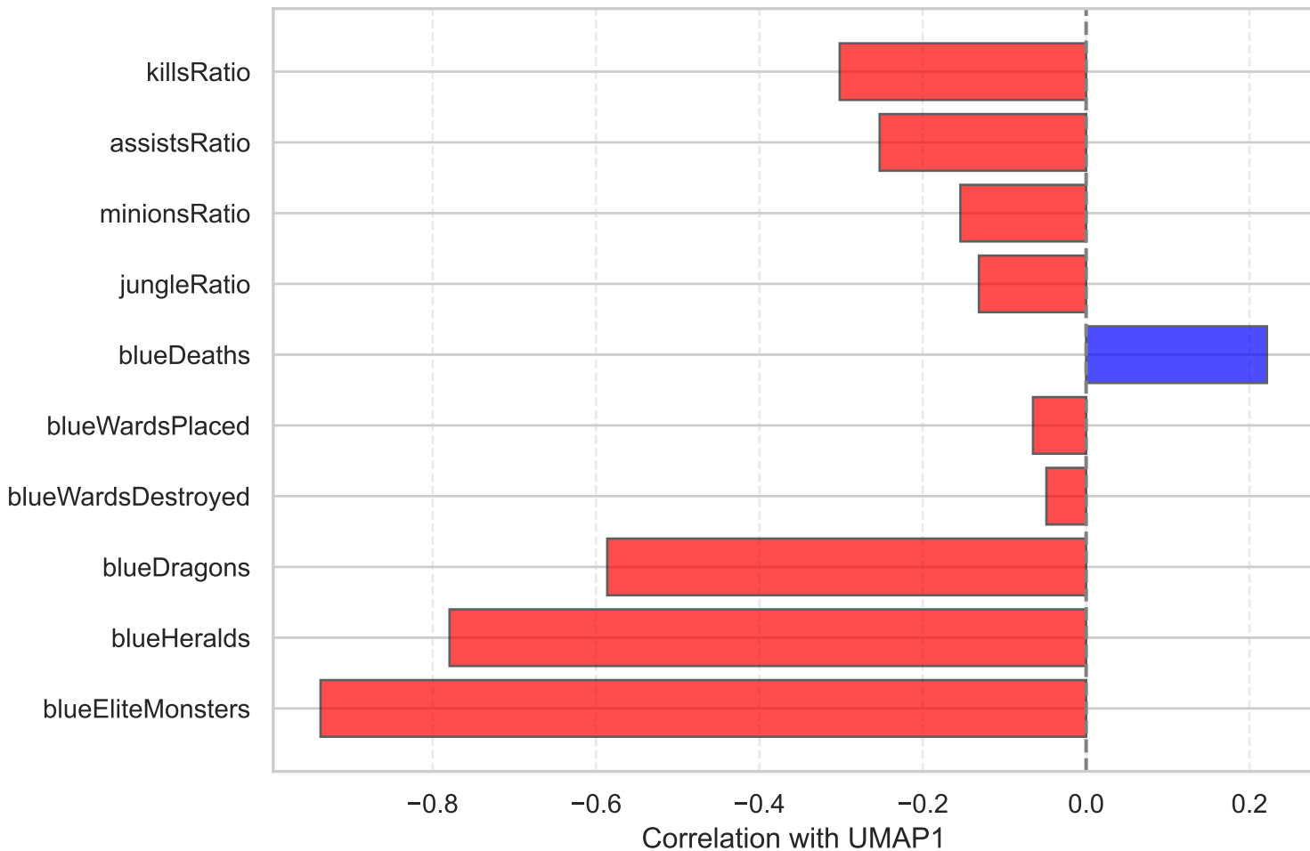
Correlations UMAP1 UMAP Feature Correlations - UMAP1
