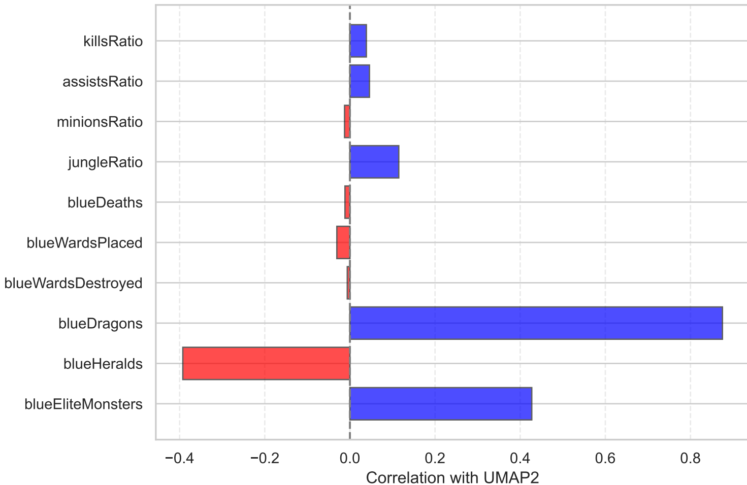
Correlations UMAP2 UMAP Feature Correlations - UMAP2
