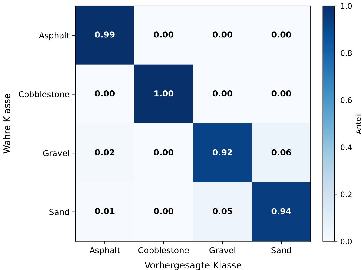
Normalisierte Konfusion Matrix – MobileNetV3 Baseline (Testset, 52.503 Patches)
