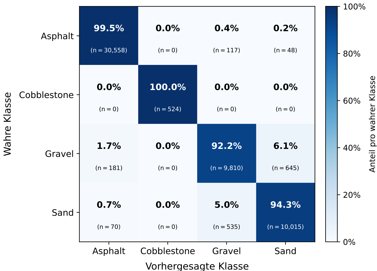
Normalisierte Konfusionsmatrix – MobileNetV3-Small Baseline (Testset, 52 503 Patches)
