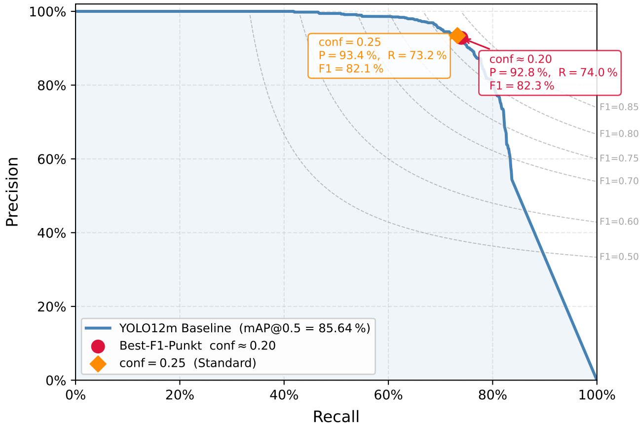
Precision-Recall-Kurve - YOLO12m Baseline (Validierungsset, 495 Bilder, IoU@0.5)
