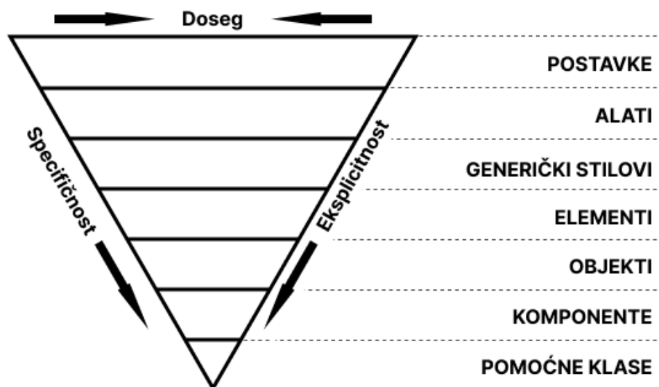
Slika 5: Prikaz arhitekture obrnutog trokuta CSS-a (Izvor: slika je rekreirana prema slici sa https://www.xfive.co/blog/itcss-scalable-maintainable-css-architecture , pristupljeno: 26.6.2026.)
