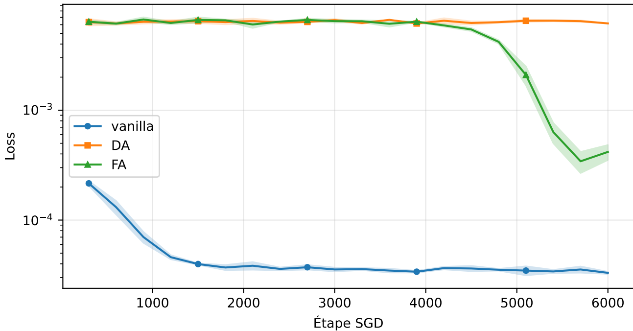
Loss vs étapes SGD — NN classique, setup UV, N=300
