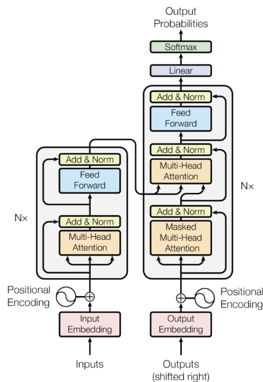
Ilustración 1 - Esquema modelo Transformers
