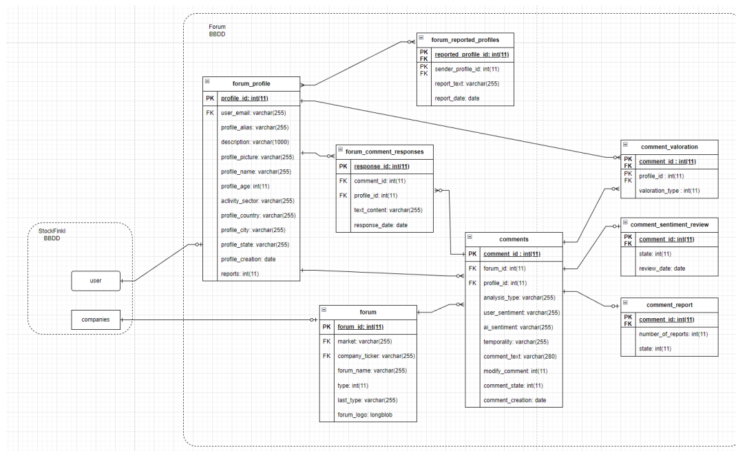
Ilustración 39 - Diagrama Entidad-Relación de base de datos
