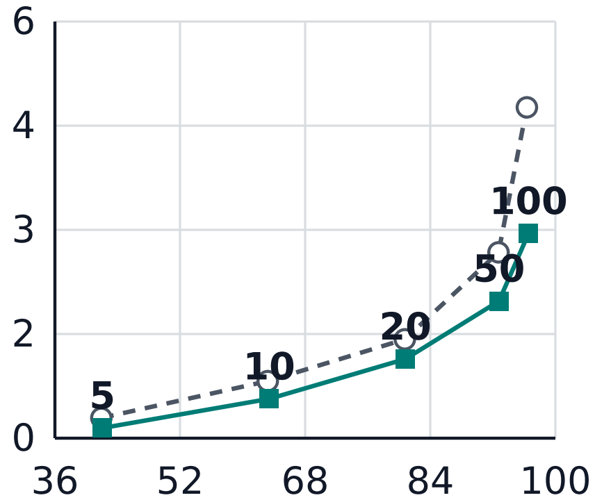
(a) VL-SAT
