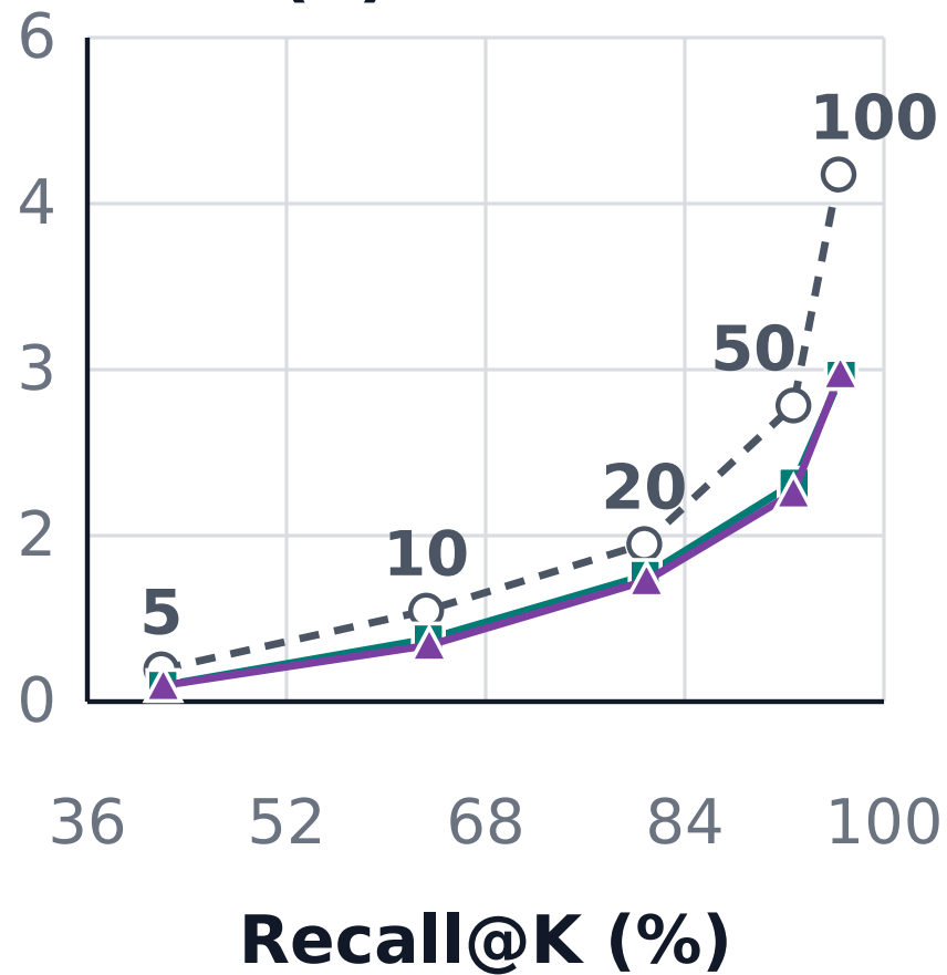
(a) VL-SAT
