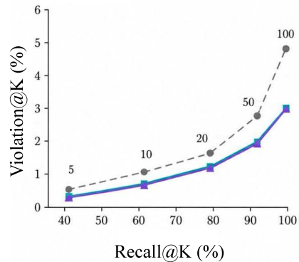
(a) VL-SAT
