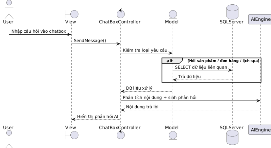
Hình 3.7 Sơ đồ Sequence Diagram chức năng Chatbox AI
