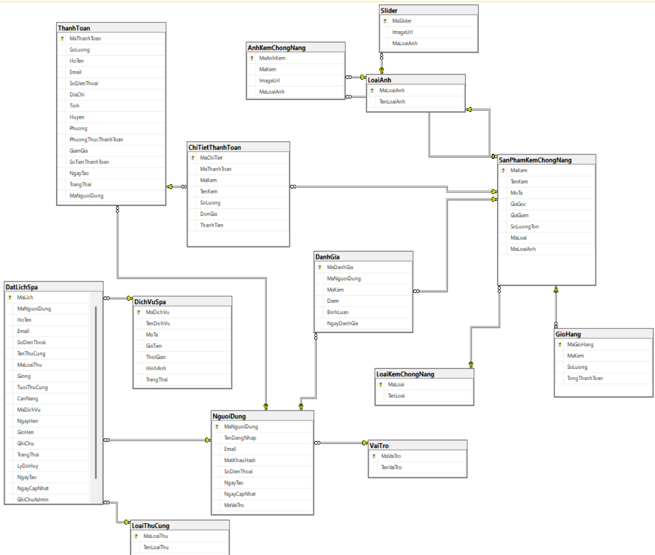
Hình 3.3 Sơ đồ cơ sở dữ liệu
