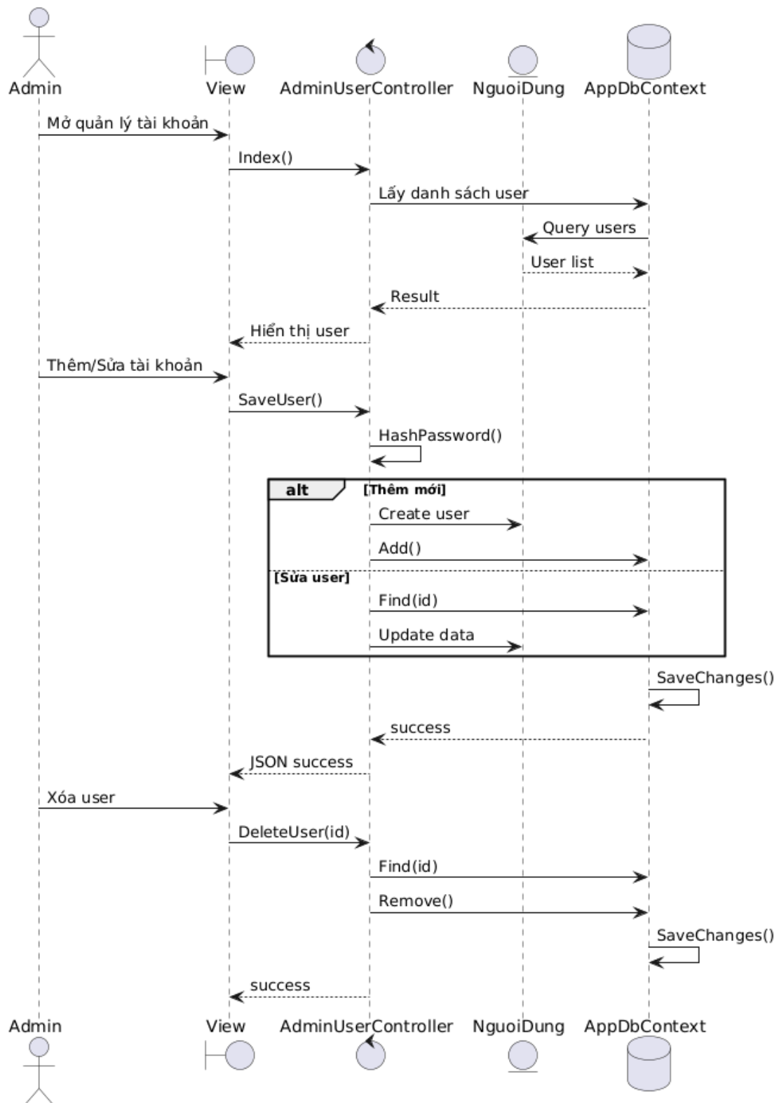
Hình 3.6 Sơ đồ Sequence Diagram quản lý tài khoản
