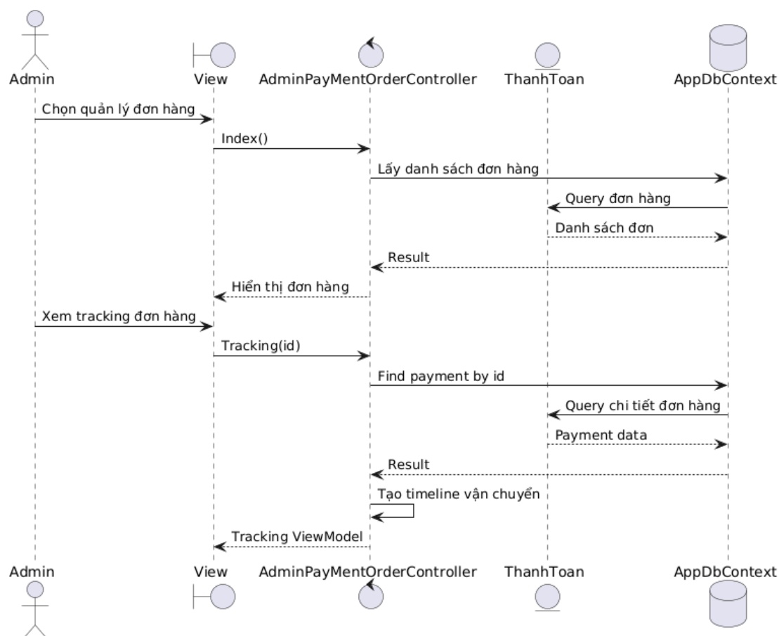
Hình 3.6 Sơ đồ Sequence Diagram quản lý đơn hàng
