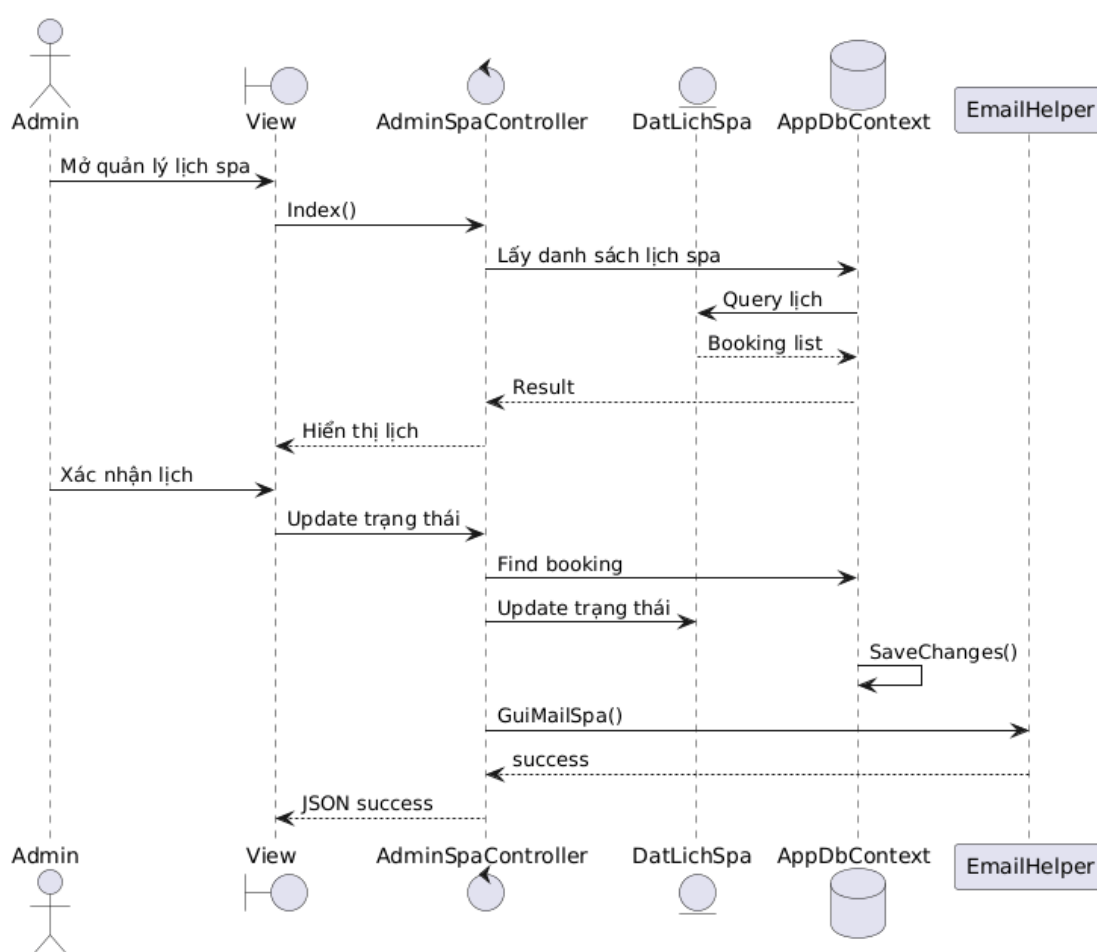
Hình 3.7 Sơ đồ Sequence Diagram quản lý spa
