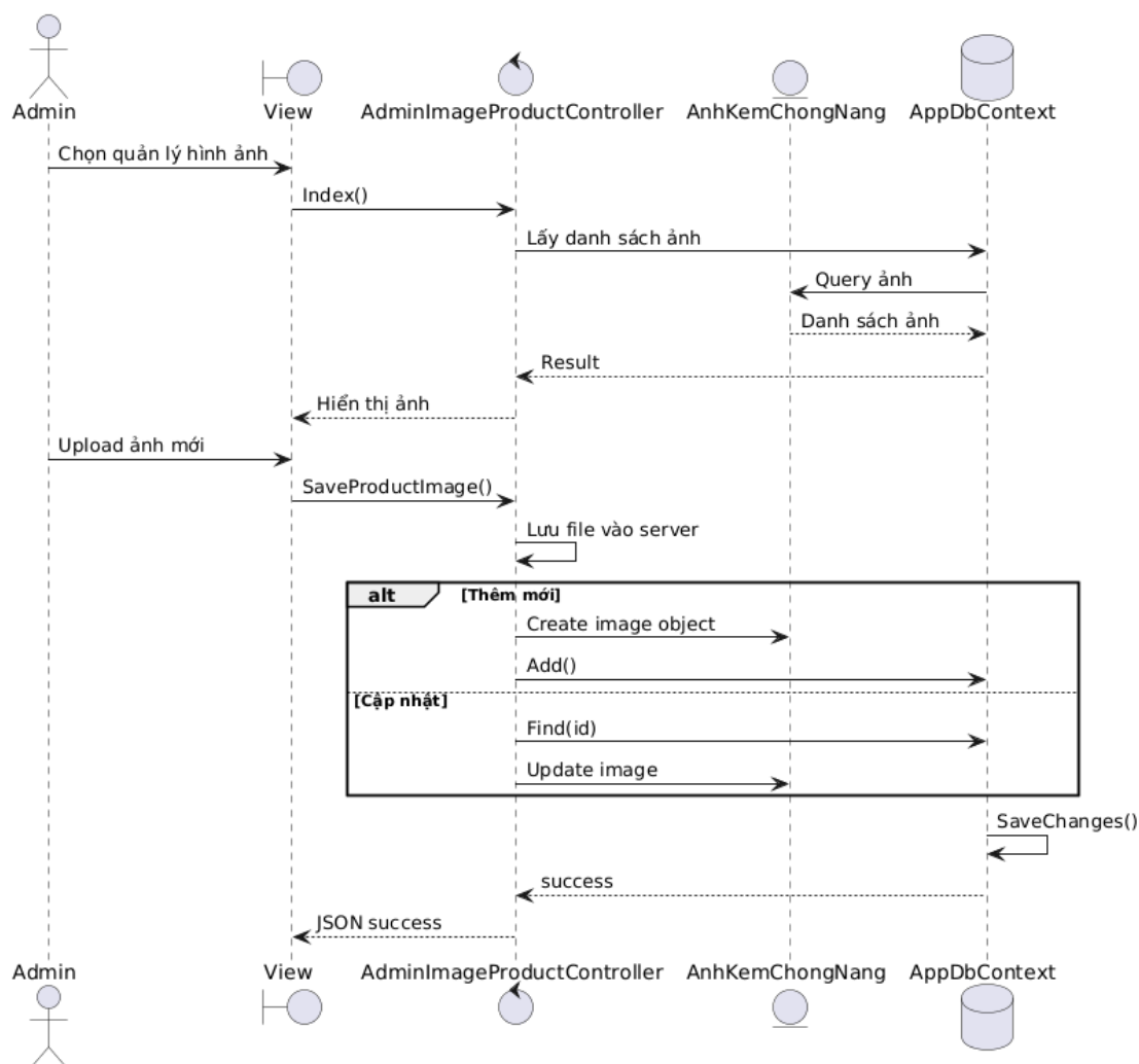
Hình 3.5 Sơ đồ Sequence Diagram quản lý hình ảnh
