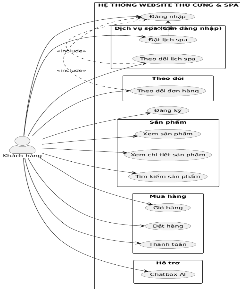
Hình 3.2. Usecase của tác nhân khách hàng
