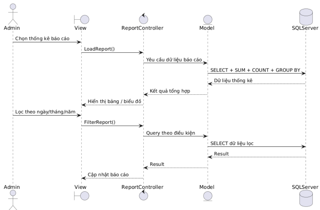
Hình 3.7 Sơ đồ Sequence Diagram chức năng thống kê báo cáo
