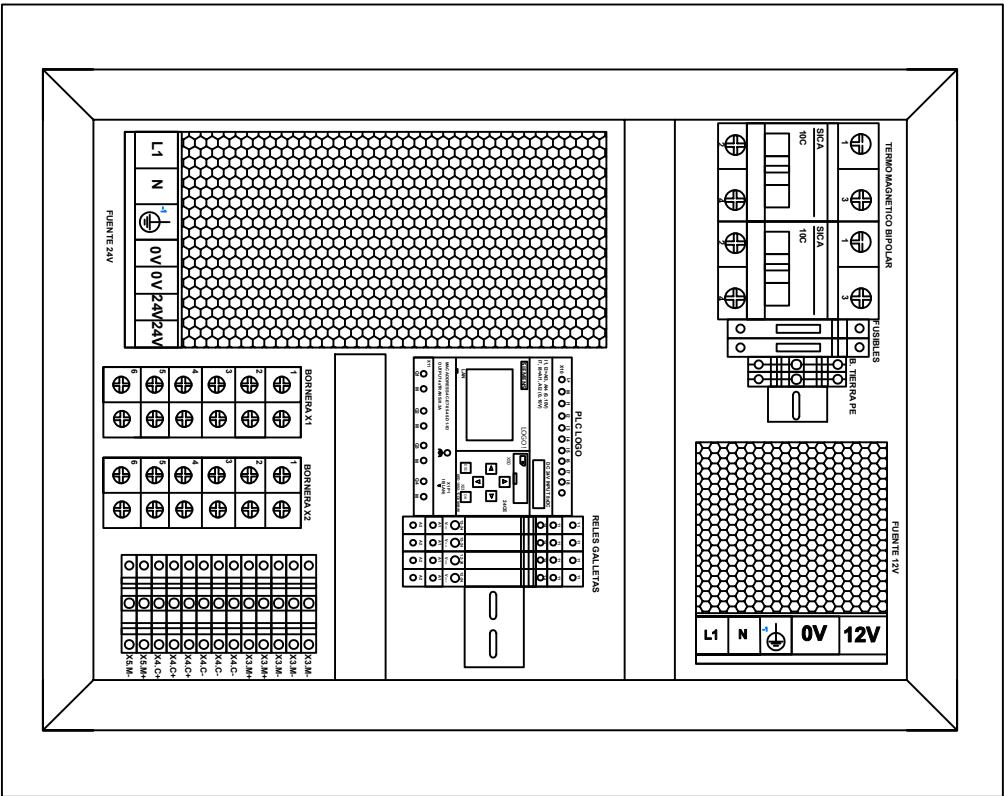
VISTA INTERIOR DEL TABLERO
