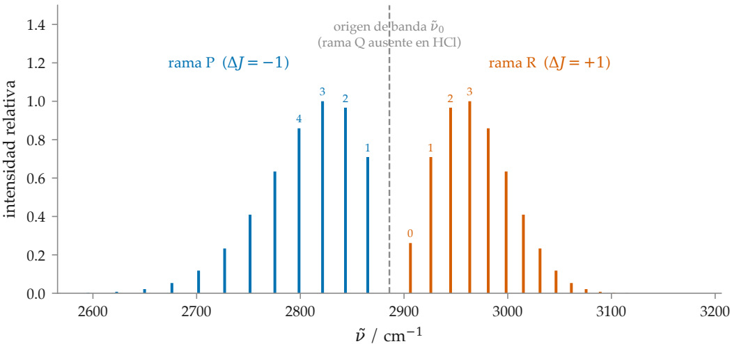
Espectro roto-vibracional del HCl ( \nu = 0 \rightarrow 1 ): la intensidad sigue la población de Boltzmann
